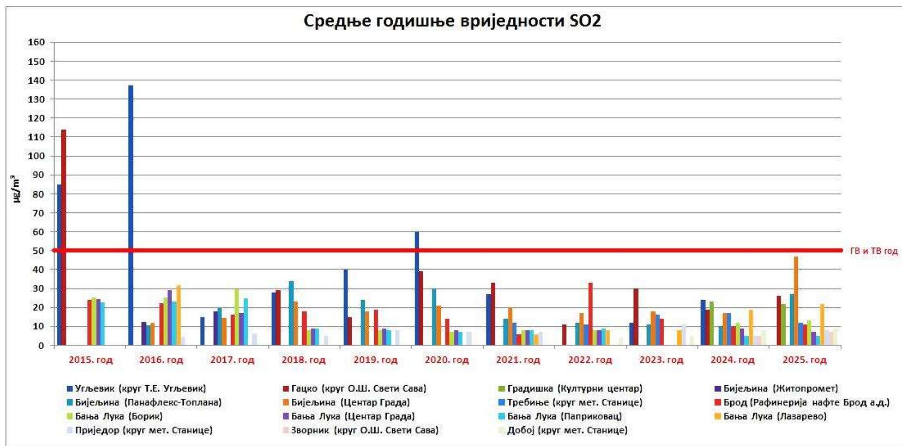
Графикон 2. Упоредни приказ средњих годишњих концентрације SO 2 µg/m 3 по мјерним мјестима и годинама.
