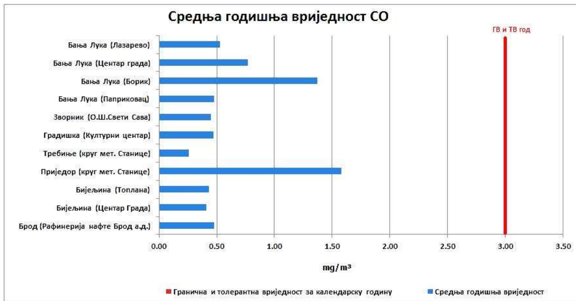
Графикон 31. Упоредни приказ средње годишње концентрације CO mg/m³ по мјерним мјестима у 2025. години
