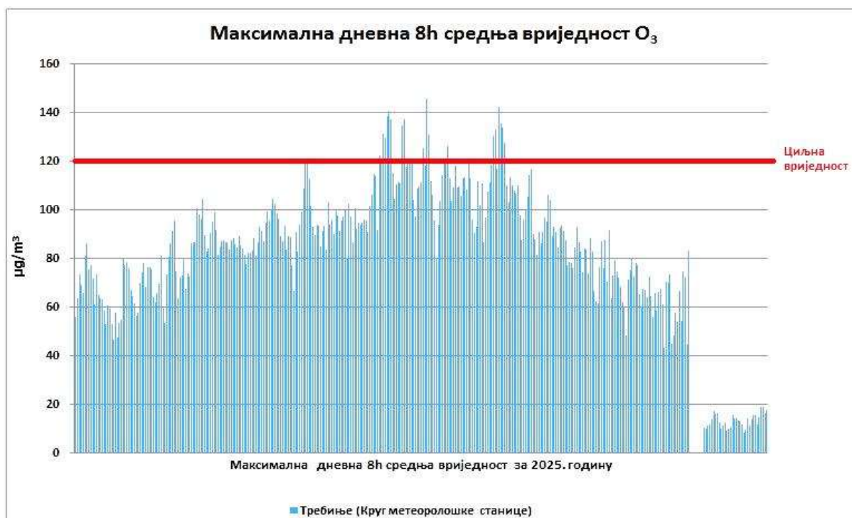
Графикон 40. Приказ максималних дневних осмосмочасовних средњих вриједности приземног озона O_3 \mu g/m^3 Требиње М.М. круг мет. станице у 2025. години
