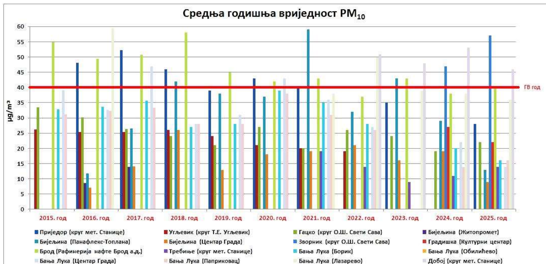
Графикон 18. Упоредни приказ средњих годишњих концентрације PM_{10} \mu g/m^3 по мјерним мјестима и годинама
