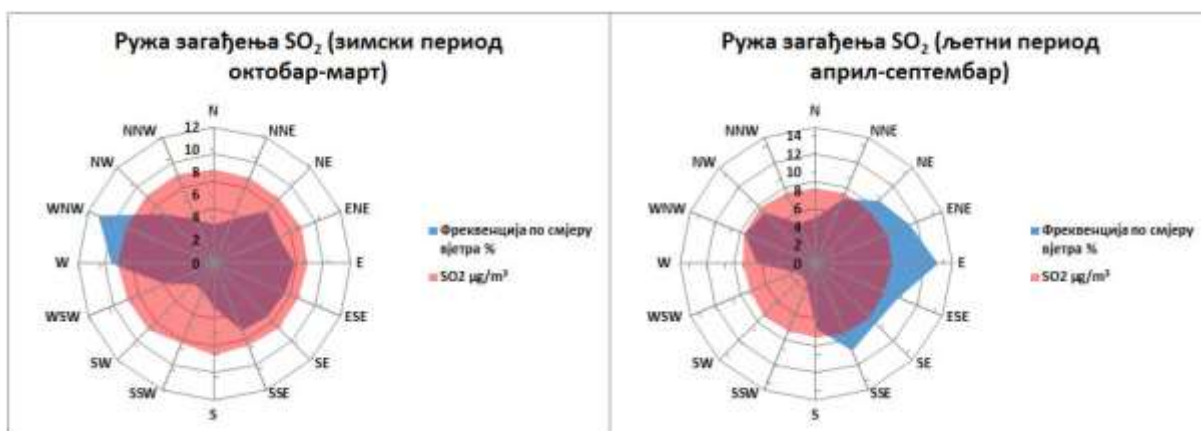
Графикон 8. Ружа загађења \text{SO}_2 \mu\text{g}/\text{m}^3 Приједор М.М. круг мет. станице 2025. године
