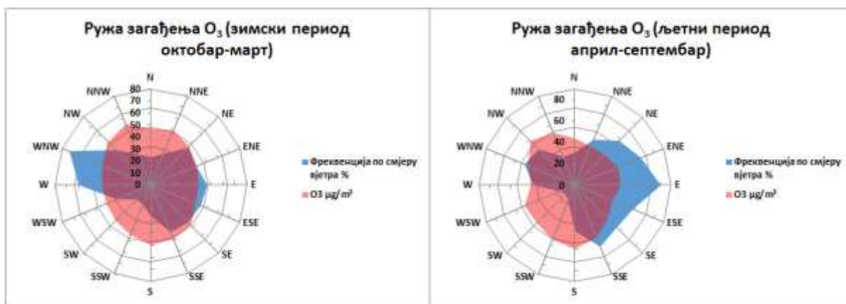
Графикон 46. Руже загађења O_3 \mu g/m^3 Приједор М.М. круг мет. станице 2025. године
