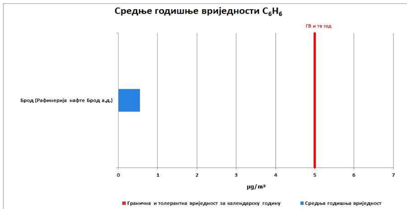
Графикон 52. Приказ средње годишње концентрације C 6 H 6 µg/m 3 по мјерним мјестима у 2025. години.
