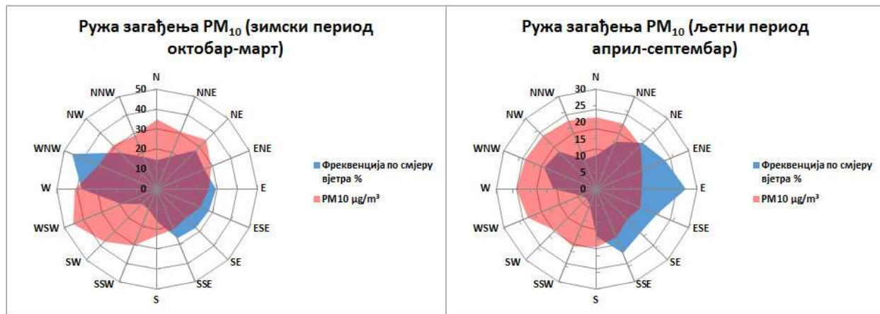
Графикон 24. Руже загађења PM_{10} \mu g/m^3 Приједор М.М. круг мет. станице 2025. године
