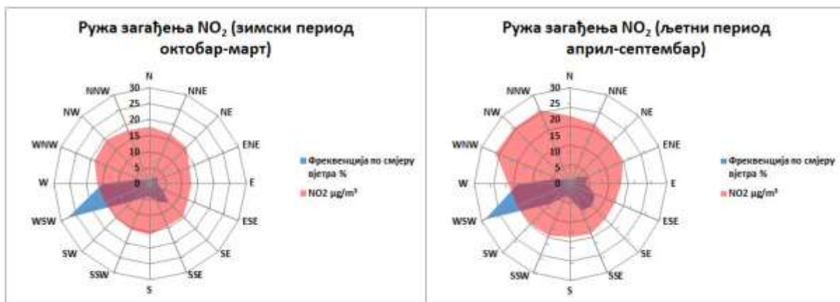
Графикон 13. Руже загађења NO 2 µg/m 3 Добој М.М. круг мет. станице 2025. године
