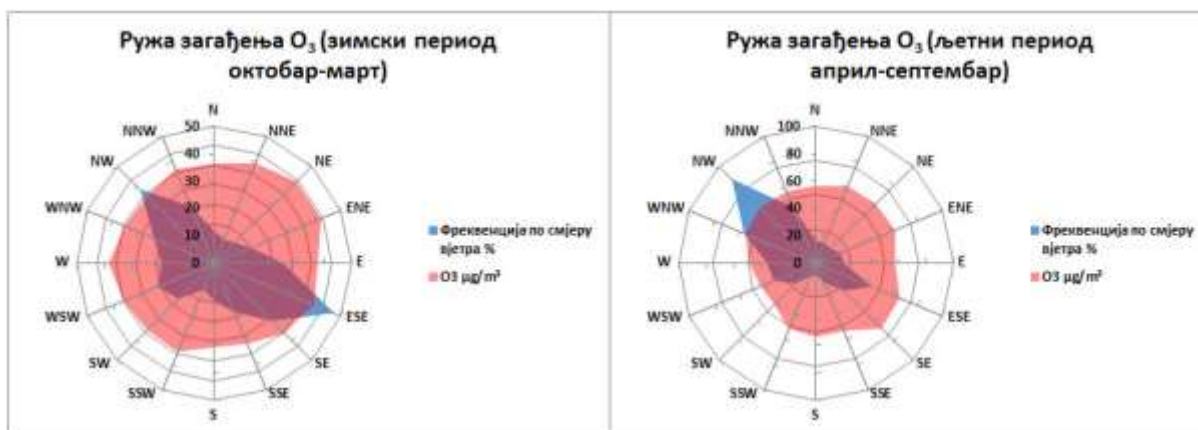
Графикон 42. Руже загађења O_3 \mu g/m^3 Брод М.М. Рафинерија нафте Брод а.д. 2025. године
