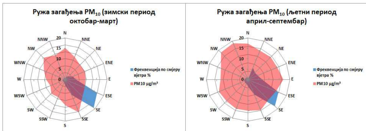
Графикон 23. Руже загађења PM_{10} \mu g/m^3 Требиње М.М. круг мет. станице 2025. Године
