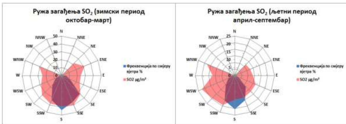
Графикон 5. Руже загађења SO 2 µg/m 3 Гацко М.М. круг О.Ш. Свети Сава 2025. године
