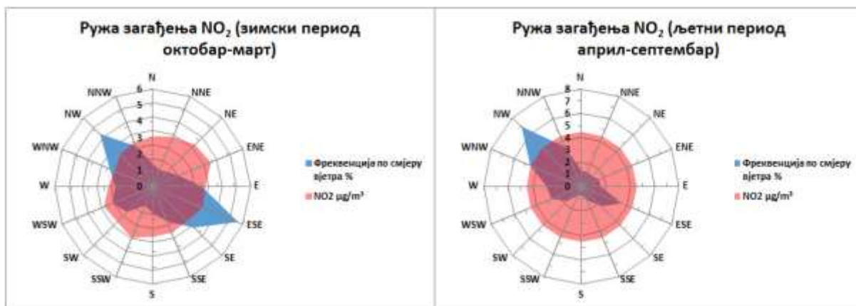
Графикон 11. Ружа загађења \text{NO}_2 \mu\text{g}/\text{m}^3 Брод М.М. Рафинерија нафте Брод а.д. 2025. године
