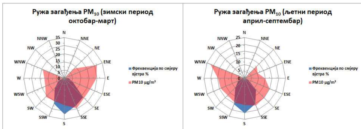
Графикон 20. Ружа загађења PM_{10} \mu g/m^3 Гацко М.М. круг О.Ш. "Свети Сава" 2025. године
