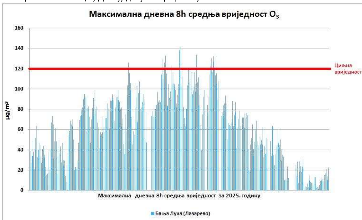
Графикон 39. Приказ максималних дневних осмосмочасовних средњих вриједности приземног озона O_3 \mu g/m^3 Бања Лука М.М. Лазарево у 2025. години
