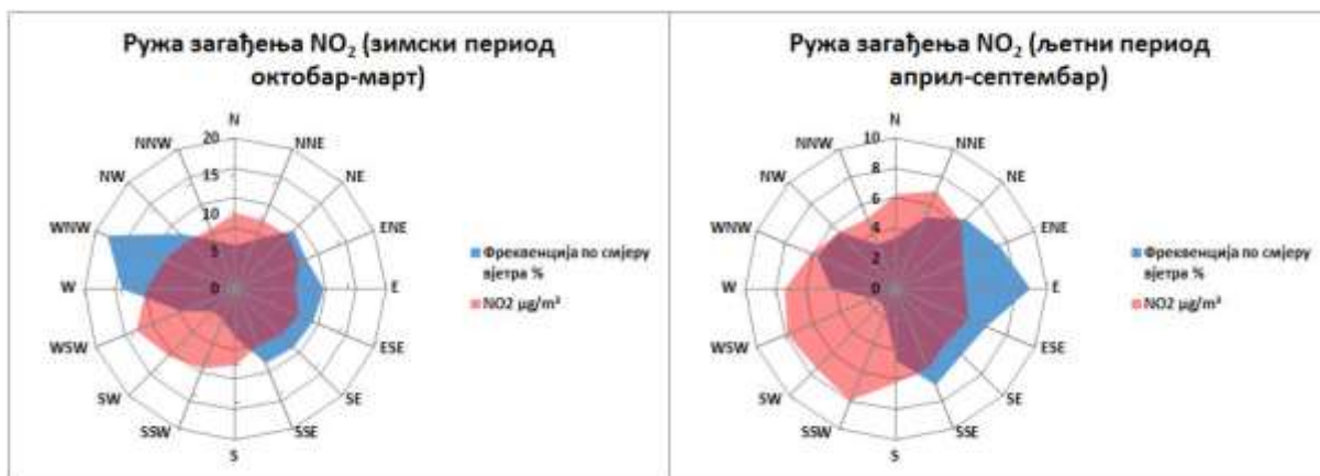
Графикон 16. Руже загађења \text{NO}_2 \mu\text{g}/\text{m}^3 Приједор М.М. круг мет. станице 2025. године
