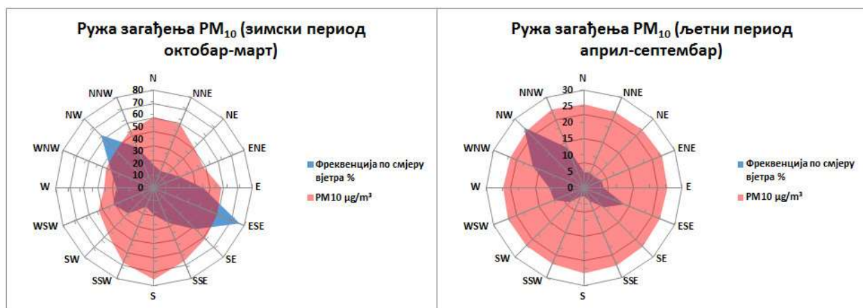
Графикон 19. Ружа загађења PM_{10} \mu g/m^3 Брод М.М. Рафинерија нафте Брод а.д. 2025. године
