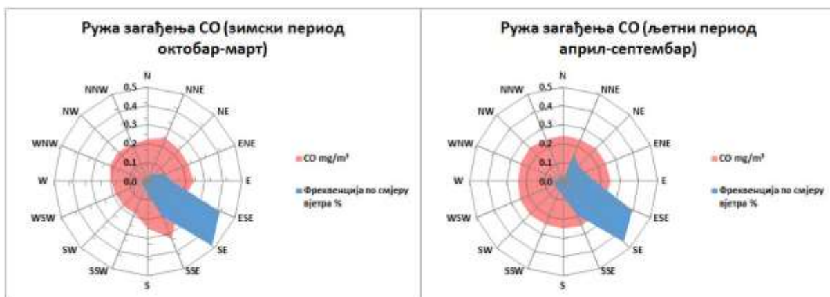
Графикон 36. Руже загађења CO mg/m 3 Требиње М.М. круг мет. станице 2025. године
