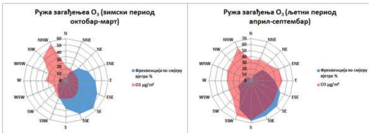
Графикон 44. Руже загађења O_3 \mu g/m^3 Бања Лука М.М. Лазаарево 2025. године
