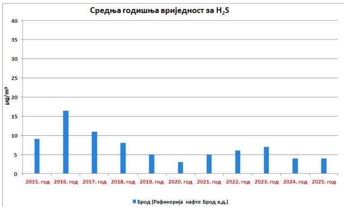
Графикон 50. Упоредни приказ средње годишње концентрације водоник сулфида \mu\text{g}/\text{m}^3 на мјерном мјесту Рафинерија нафте Брод а.д. у Броду по годинама.
