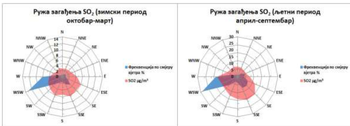
Графикон 4. Руже загађења \text{SO}_2 \mu\text{g}/\text{m}^3 Добој М.М. круг мет. станице 2025. године
