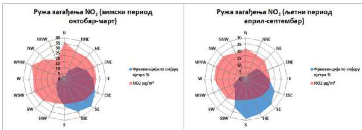
Графикон 14. Руже загађења NO 2 µg/m 3 Бања Лука М.М. Лазарево 2025. године
