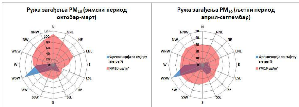
Графикон 21. Руже загађења PM_{10} \mu g/m^3 Добој М.М. круг мет. станице 2025. године
