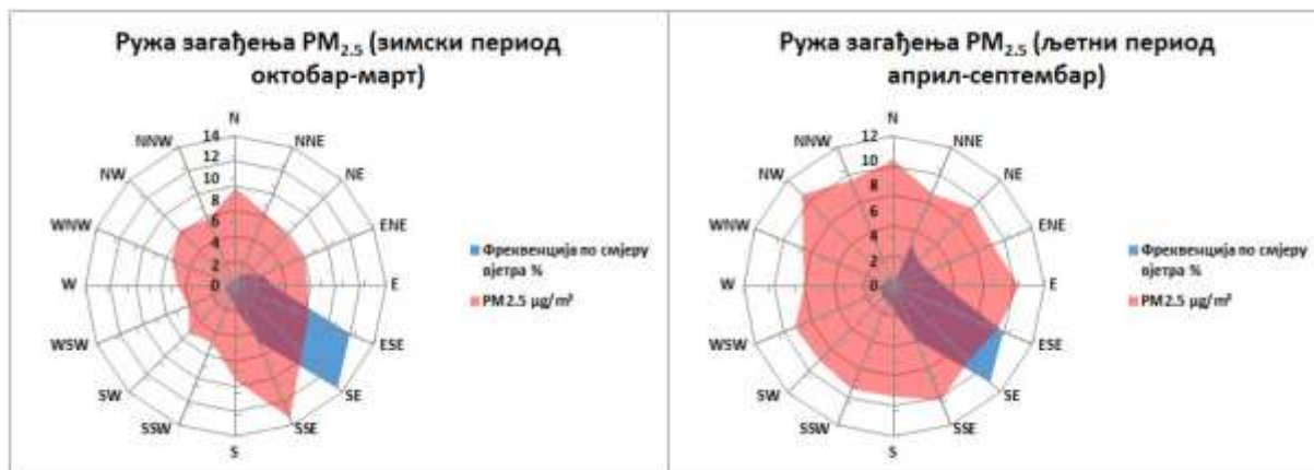
Графикон 29. Руже загађења PM_{2.5} \mu g/m^3 Требиње М.М. круг мет. станице 2025. године
