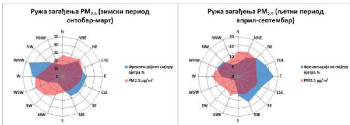
Графикон 30. Руже загађења PM_{2.5} \mu g/m^3 Приједор М.М. круг мет. станице 2025. године
