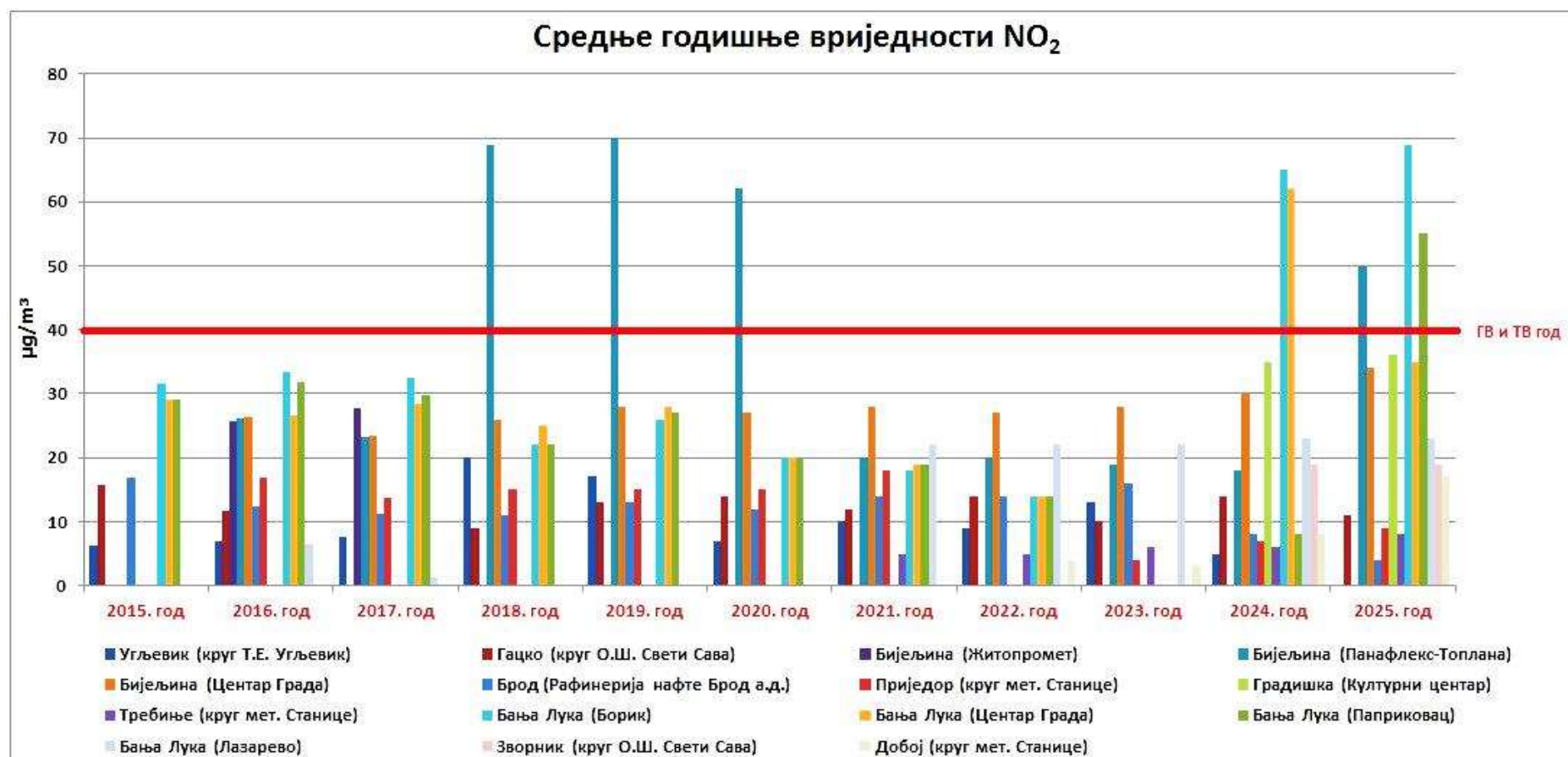
Графикон 10. Упоредни приказ средњих годишњих концентрације NO 2 µg/m 3 по мјерним мјестима и годинама
