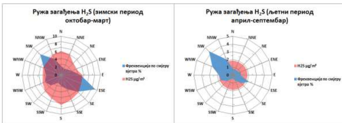
Графикон 51. Руже загађења H 2 S \mu\text{g}/\text{m}^3 Брод М.М. Рафинерија нафте Брод а.д. 2025. године
