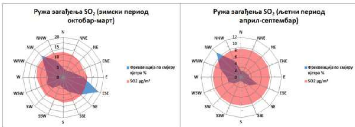
Графикон 3. Руже загађења \text{SO}_2 \mu\text{g}/\text{m}^3 Брод М.М. Рафинерија нафте Брод а.д. 2025. године
