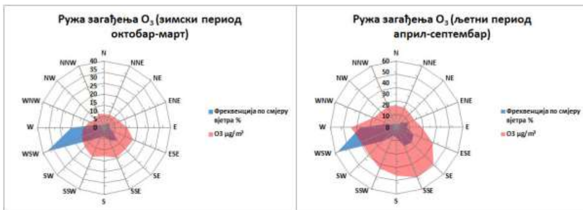
Графикон 43. Руже загађења O_3 \mu g/m^3 Добој М.М. круг мет. станице 2025. године
