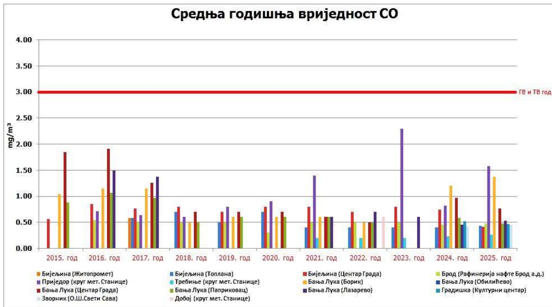
Графикон 32. Упоредни приказ средњих годишњих концентрација CO mg/m³ по мјерним мјестима и годинама
