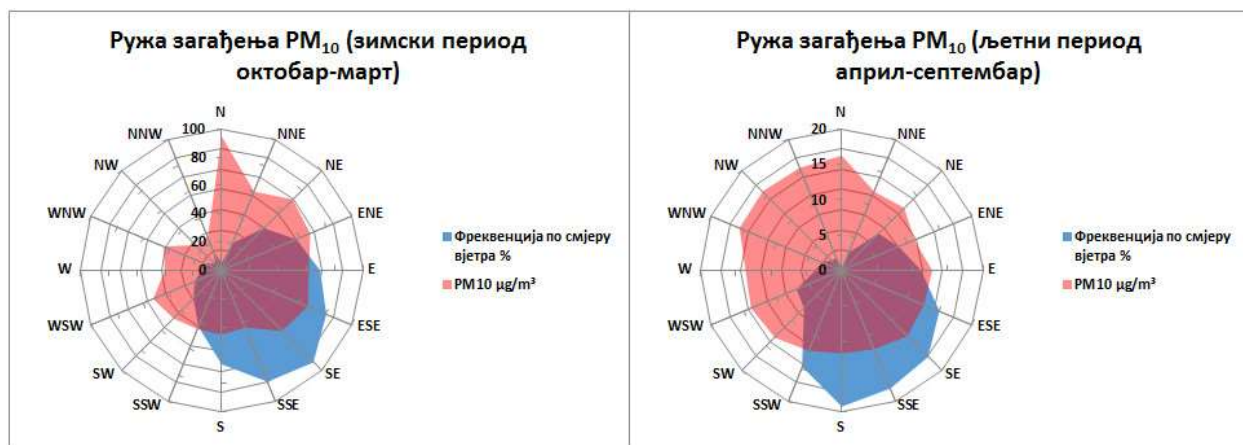
Графикон 22. Руже загађења PM_{10} \mu g/m^3 Бања Лука М.М. Лазарево 2025. године
