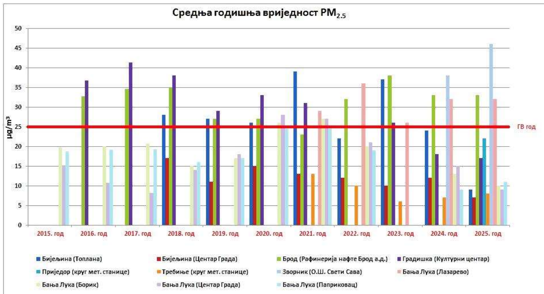
Графикон 26. Упоредни приказ средњих годишњих концентрације PM_{2.5} \mu g/m^3 по мјерним мјестима и годинама.
