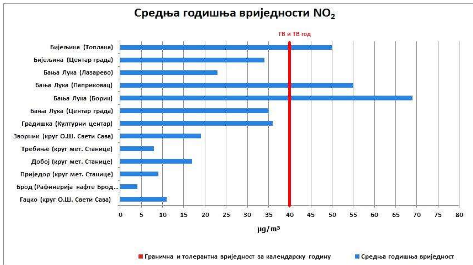
Графикон 9. Упоредни приказ средње годишње концентрације NO 2 µg/m³ по мјерним мјестима у 2025. години
