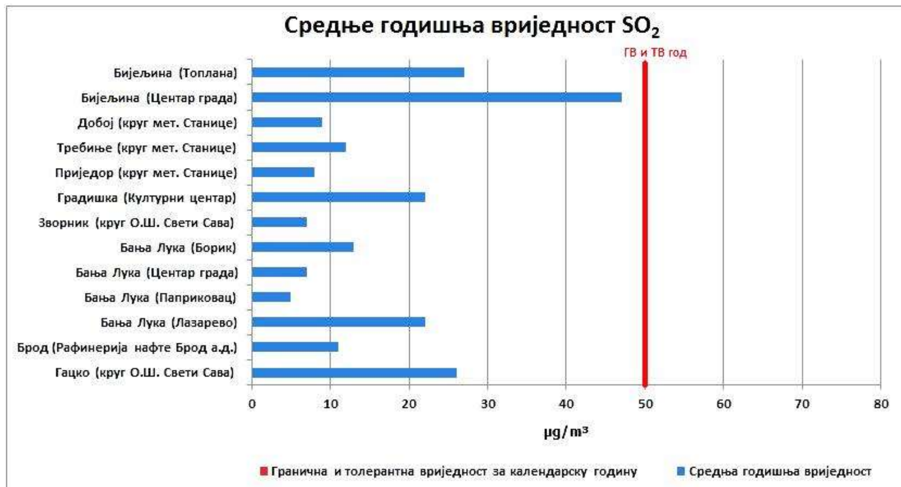
Графикон 1. Упоредни приказ средње годишње концентрације SO 2 µg/m³ по мјерним мјестима у 2025. години.
