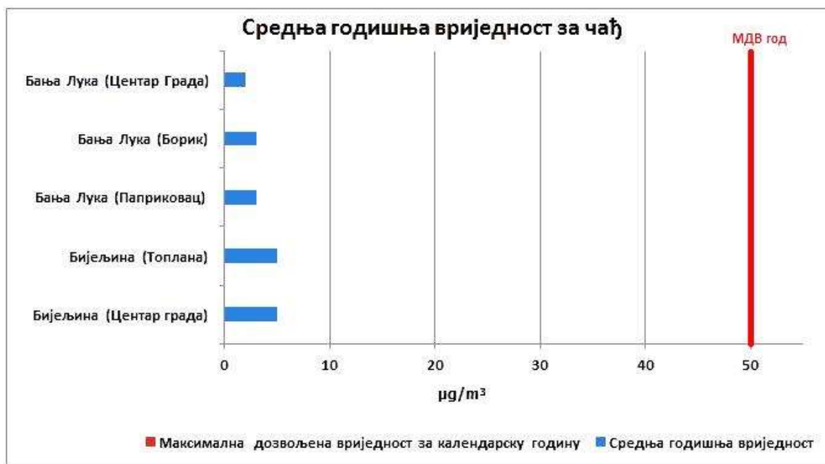
Графикон 47. Упоредни приказ средње годишње концентрације чађи µg/m³ по мјерним мјестима у 2025. години.
