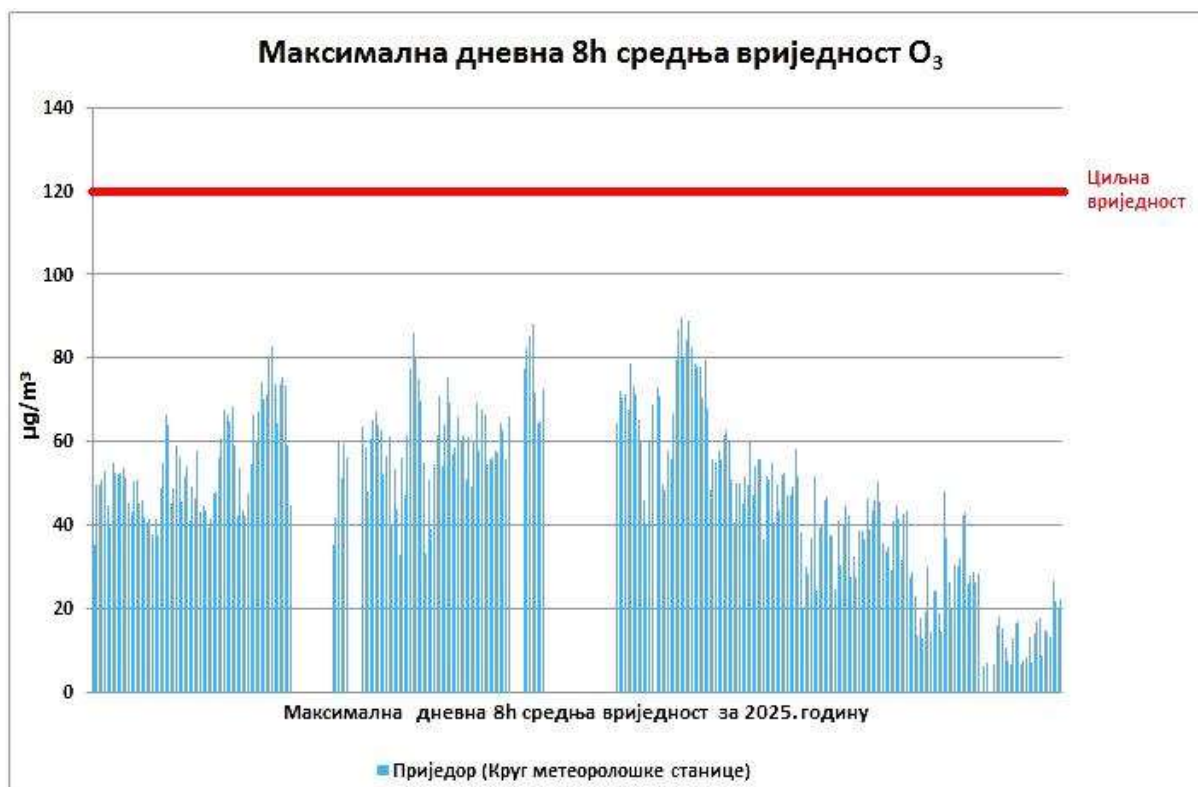
Графикон 41. Приказ максималних дневних осмосочасовних средњих вриједности приземног озона O_3 \mu g/m^3 Приједор М.М. круг мет. станице у 2025. години
