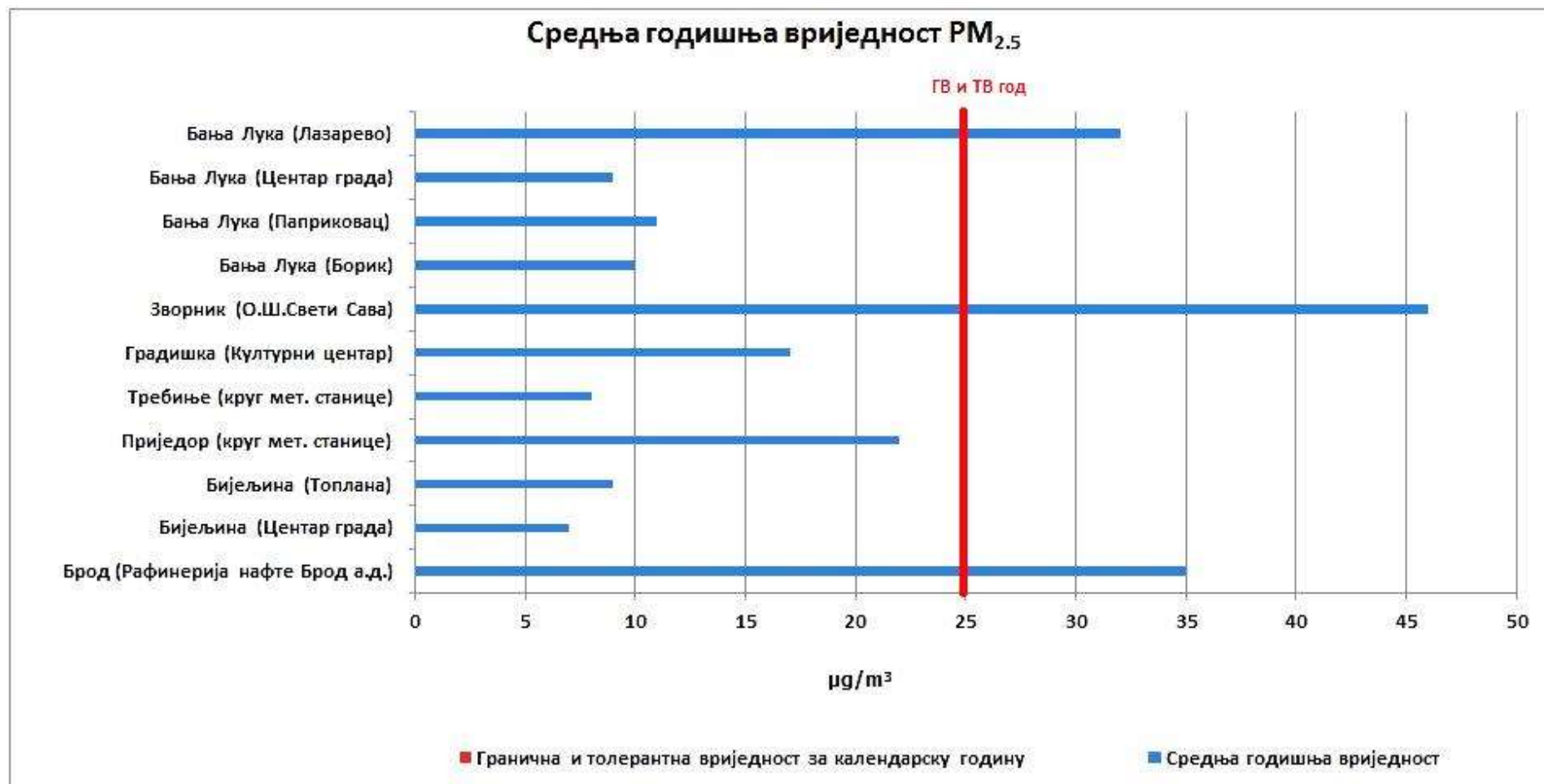
Графикон 25. Упоредни приказ средње годишње концентрације PM_{2.5} \mu g/m^3 по мјерни мјестима у 2025. години.
