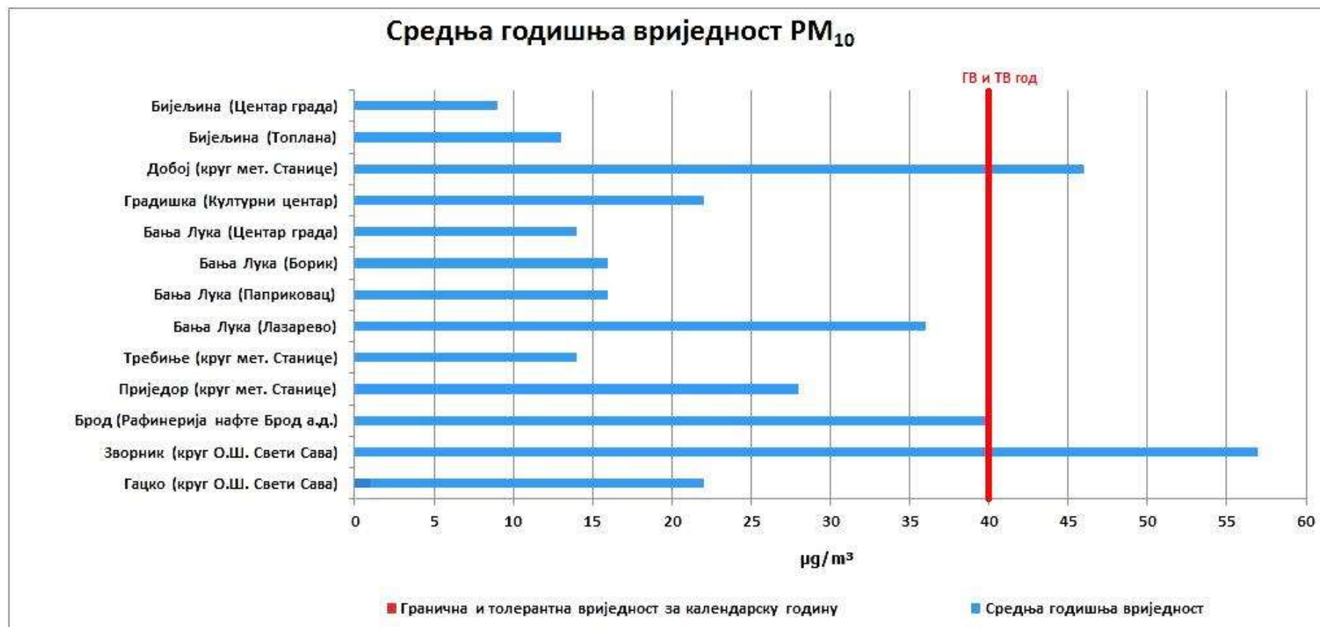
Графикон 17. Упоредни приказ средње годишње концентрације PM_{10} \mu g/m^3 по мјерним мјестима у 2025. години
