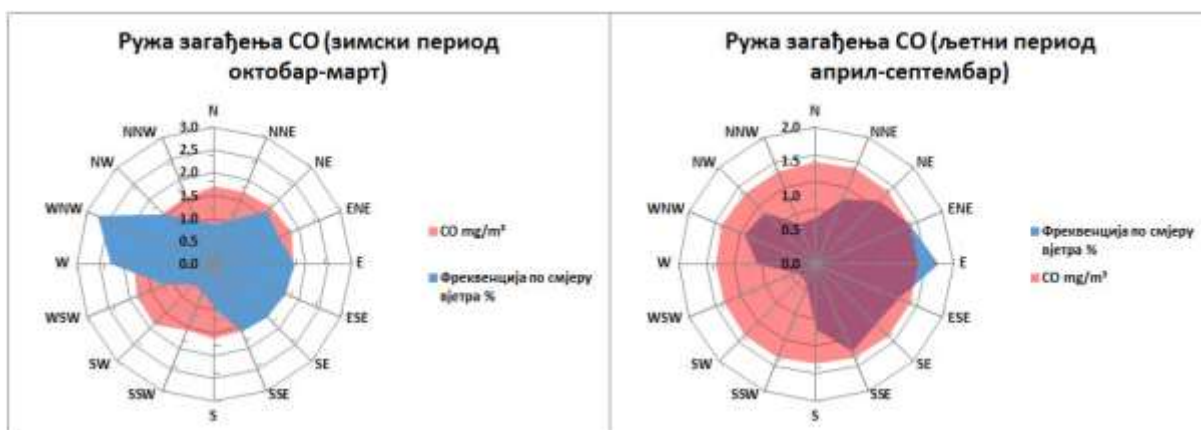
Графикон 34. Ружа загађења \text{CO mg}/\text{m}^3 Приједор М.М. круг мет. станице 2025. године
