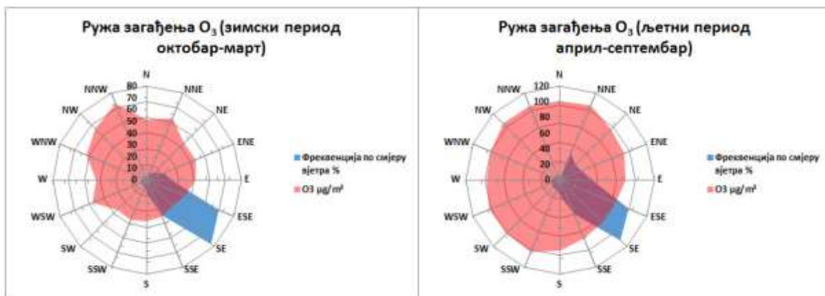
Графикон 45. Руже загађења O_3 \mu g/m^3 Требиње М.М. круг мет. станице 2025. године
