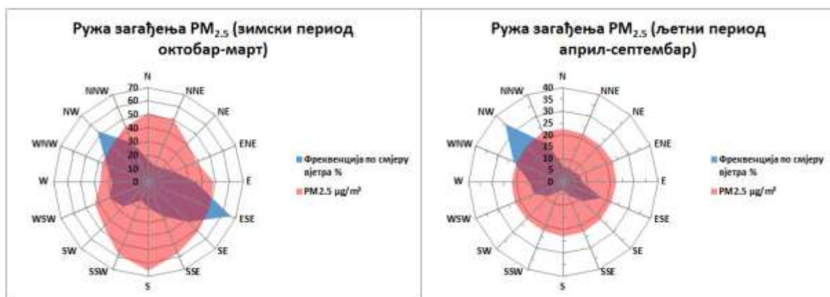
Графикон 27. Руже загађења PM_{2.5} \mu g/m^3 Брод М.М. Рафинерија нафте Брод а.д. 2025. године
