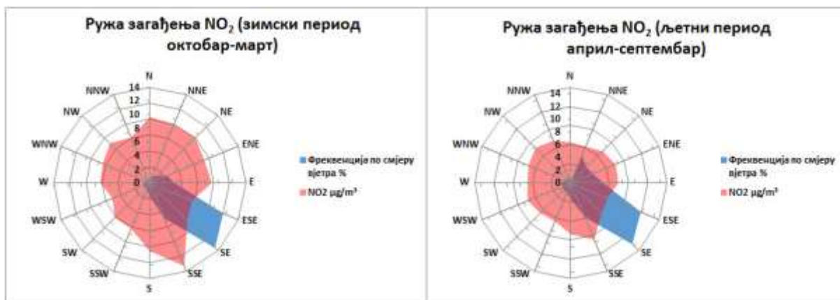
Графикон 15. Руже загађења \text{NO}_2 \mu\text{g}/\text{m}^3 Требиње М.М. круг мет. станице 2025. године
