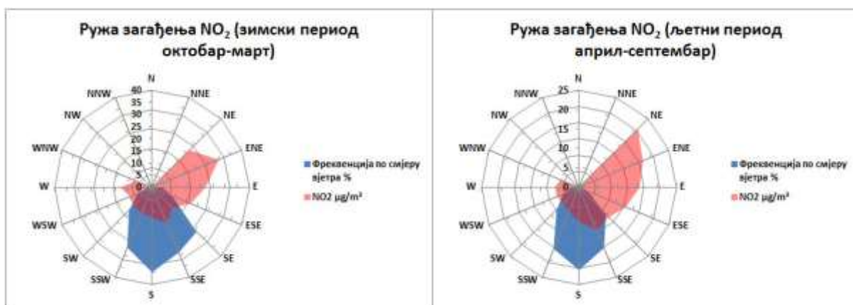
Графикон 12. Ружа загађења \text{NO}_2 \mu\text{g}/\text{m}^3 Гацко М.М. круг О.Ш. Свети Сава 2025. године
