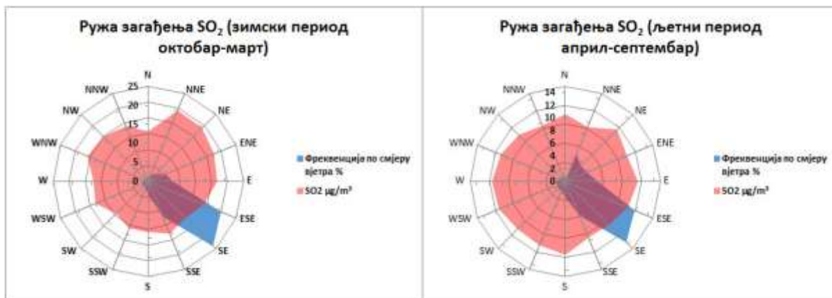
Графикон 7. Ружа загађења \text{SO}_2 \mu\text{g}/\text{m}^3 Требиње М.М. круг мет. станице 2025. године
