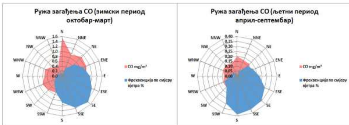
Графикон 35. Руже загађења CO mg/m 3 Бања Лука М.М. Лазарево 2025. године
