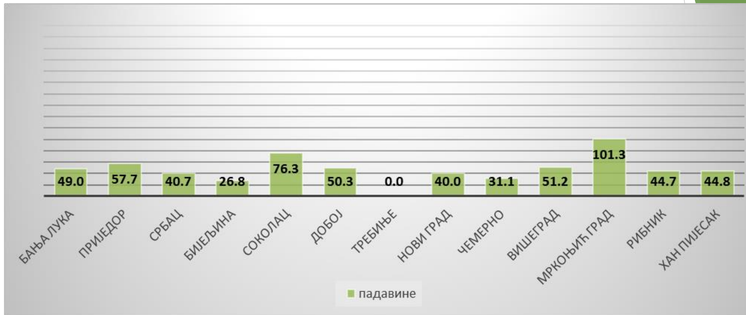
Слика 4 - Сума падавина за август 2019.године
