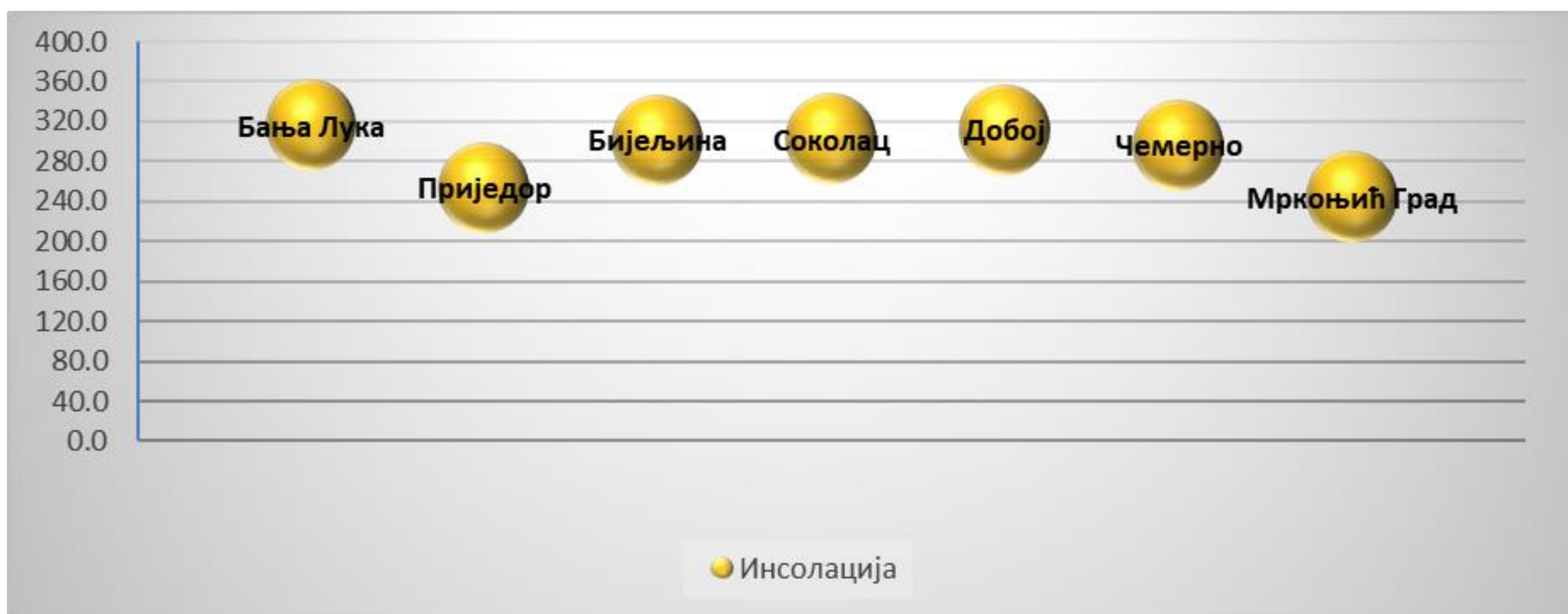
Слика 2 - Инсолација (h) за август 2019.године
