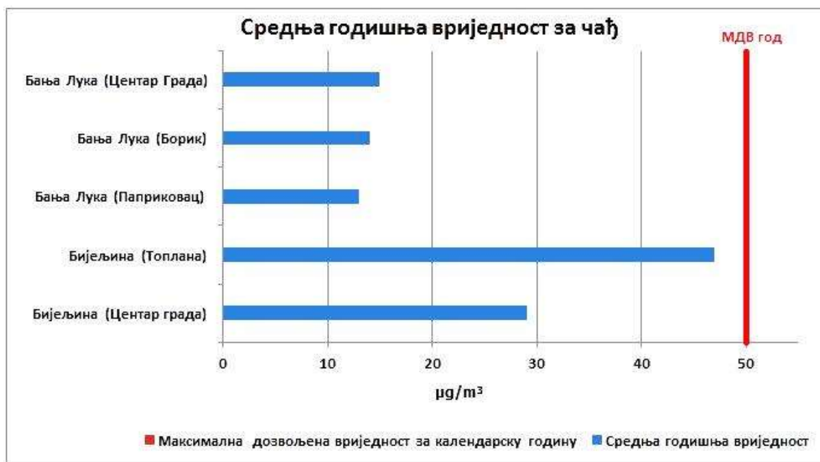
Графикон 43. Упоредни приказ средње годишње концентрације чађи µg/m³ по мјерним мјестима у 2022. години.
