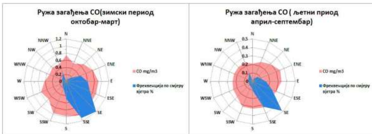
Графикон 32. Руже загађења CO mg/m 3 Добој М.М. круг мет. станице 2022. године
