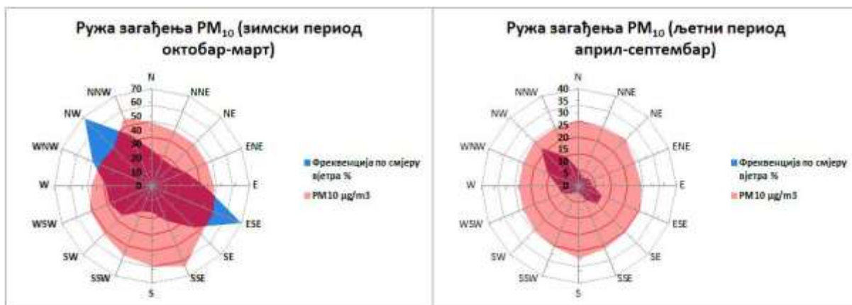
Графикон 18. Ружа загађења PM_{10} \mu g/m^3 Брод М.М. Рафинерија нафте Брод а.д. 2022. године
