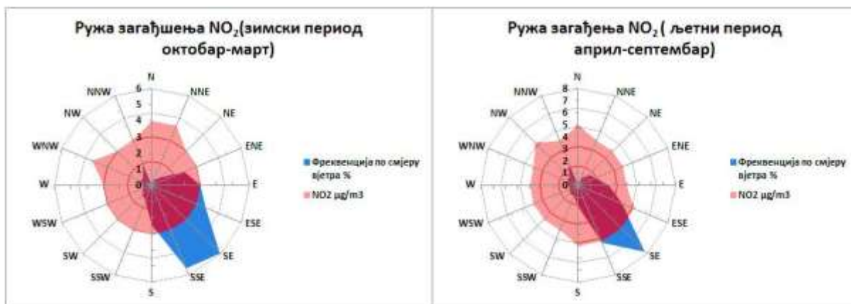
Графикон 12. Руже загађења \text{NO}_2 \mu\text{g}/\text{m}^3 Добој М.М. круг мет. станице 2022. године
