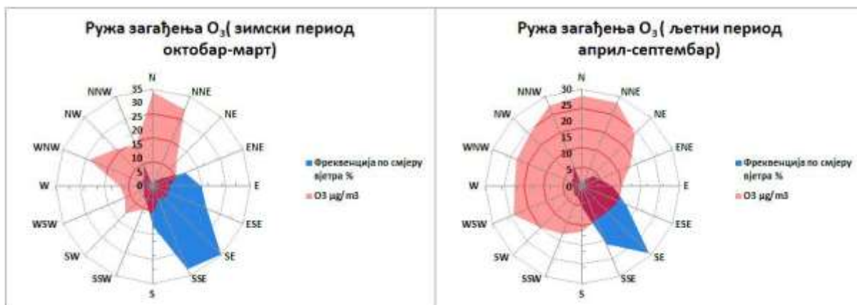
Графикон 40. Руже загађења O_3 \mu g/m^3 Добо М.М. круг мет. станице 2022. године
