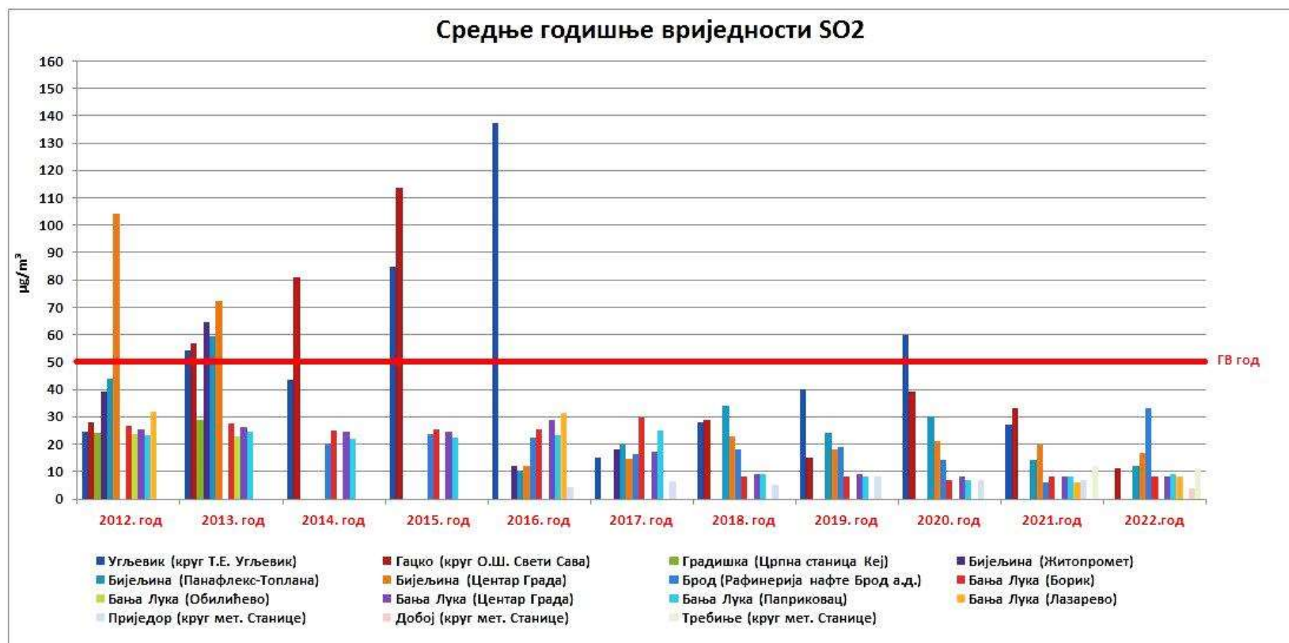
Графикон 2. Упоредни приказ средњих годишњих концентрације SO 2 \mu\text{g}/\text{m}^3 по мјерним мјестима и годинама.
