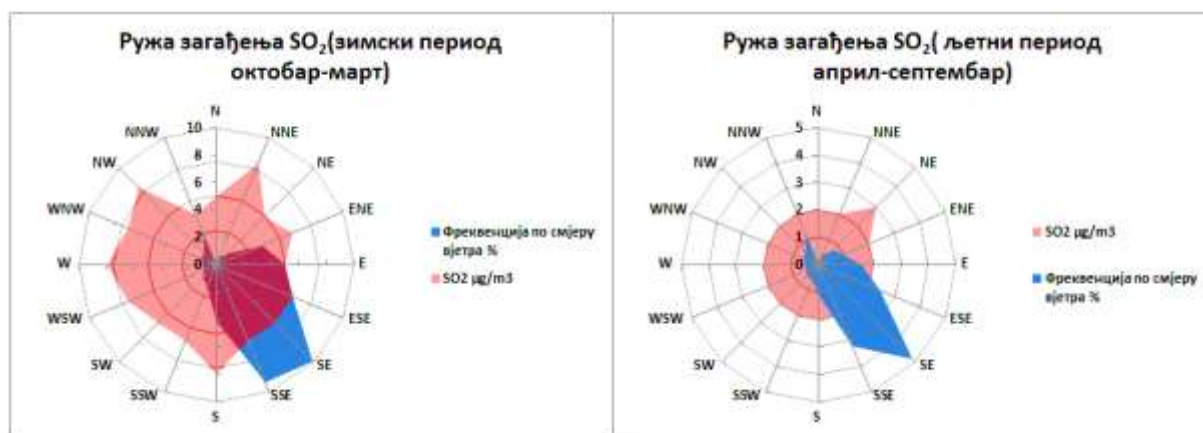
Графикон 4. Ружа загађења \text{SO}_2 \mu\text{g}/\text{m}^3 Добој М.М. круг мет. станице 2022. године
