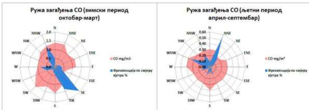
Графикон 33. Руже загађења CO mg/m³ Бања Лука М.М. Лазарево 2022. године
