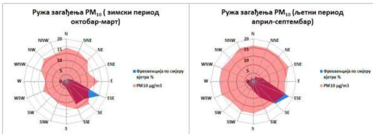
Графикон 23. Руже загађења PM_{10} \mu g/m^3 Требиње М.М. круг мет. станице 2022. године
