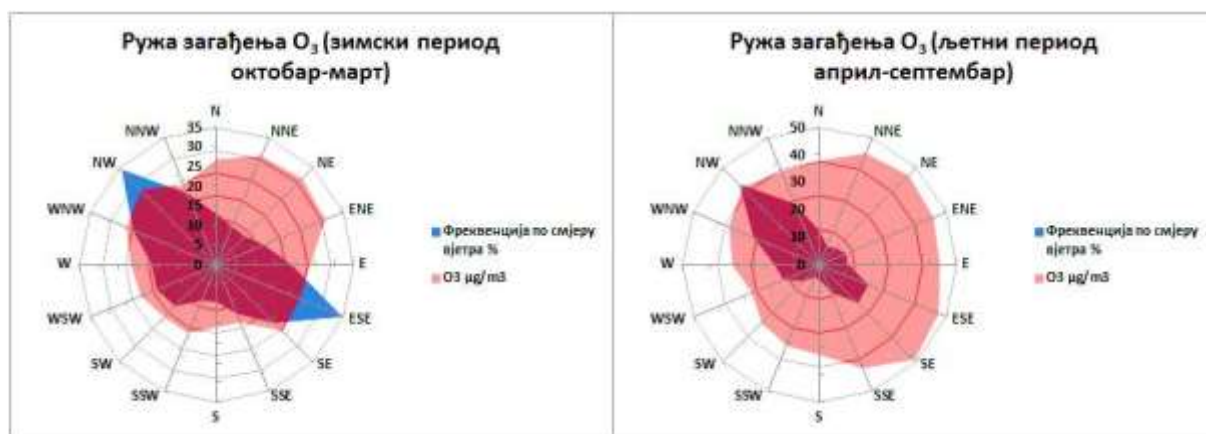
Графикон 39. Руже загађења O_3 \mu g/m^3 Брод М.М. Рафинерија нафте Брод а.д. 2022. године
