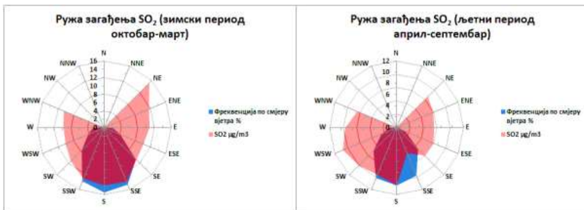
Графикон 5. Руже загађења SO 2 µg/m 3 Гацко М.М. круг О.Ш. Свети Сава 2022. године
