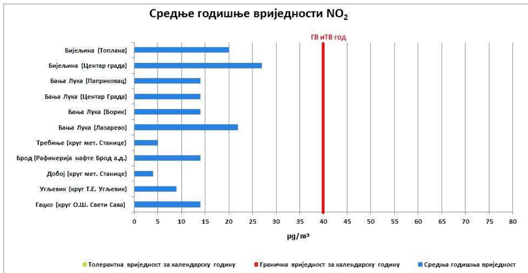
Графикон 8. Упоредни приказ средње годишње концентрације NO 2 µg/m³ по мјерним мјестима у 2022. години
