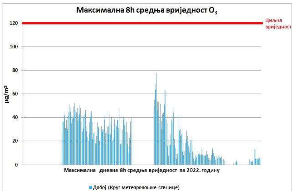
Графикон 36. Приказ максималних дневних осмосмочасовних средњих вриједности приземног озона O_3 \mu g/m^3 Добој М.М. круг мет. станице у 2022. години
