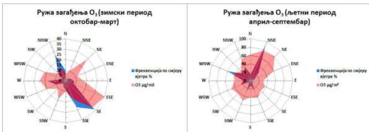
Графикон 41. Руже загађења O_3 \mu g/m^3 Бања Лука М.М. Лазаарево 2022. године
