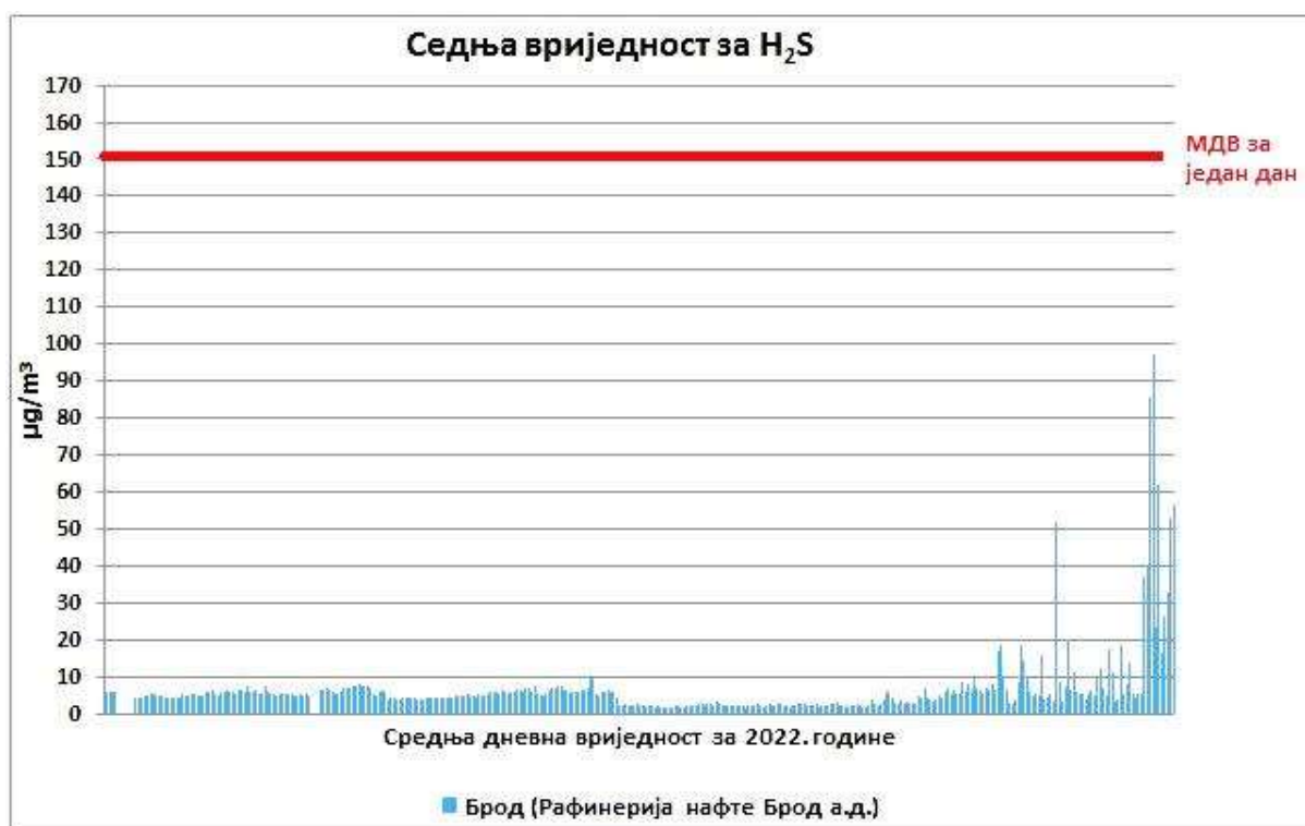
Графикон 45. Приказ средњих дневних вриједности концентрације водоник сулфида µg/m 3 у 2022. години
