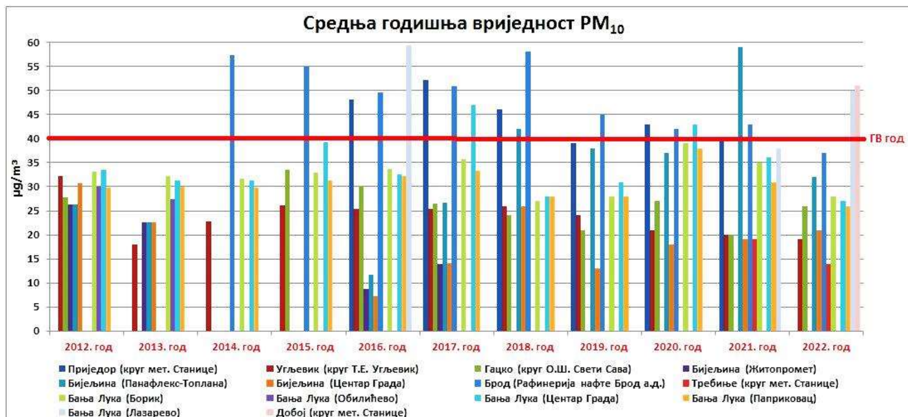
Графикон 17. Упоредни приказ средњих годишњих концентрације PM_{10} \mu g/m^3 по мјерним мјестима и годинама
