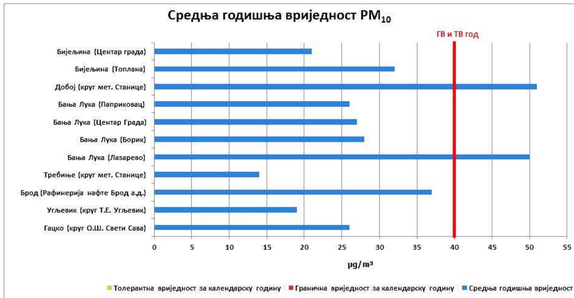
Графикон 16. Упоредни приказ средње годишње концентрације PM_{10} \mu g/m^3 по мјерним мјестима у 2022. години
