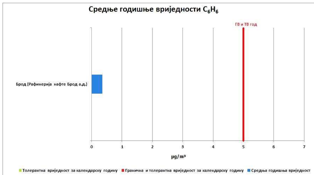
Графикон 48. Приказ средње годишње концентрације C 6 H 6 µg/m 3 по мјерним мјестима у 2022. години.
