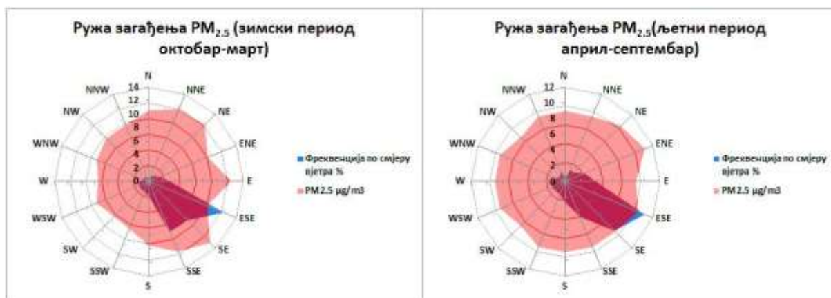
Графикон 28. Руже загађења PM_{2.5} \mu g/m^3 Требиње М.М. круг мет. станице 2022. године
