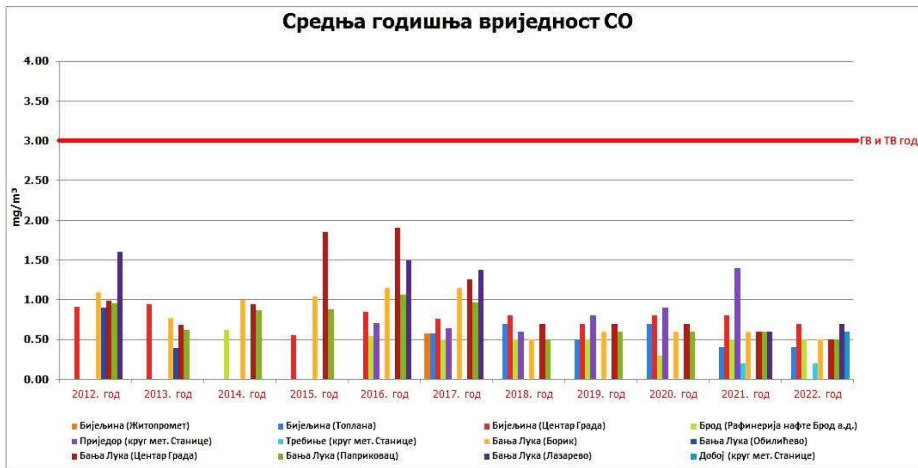
Графикон 30. Упоредни приказ средњих годишњих концентрација CO mg/m 3 по мјерним мјестима и годинама
