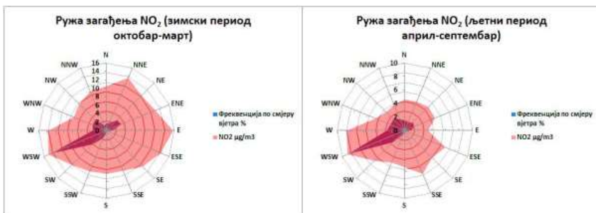
Графикон 13. Руже загађења \text{NO}_2 \mu\text{g}/\text{m}^3 Угљевик М.М. Т.Е.Угљевик 2022. године
