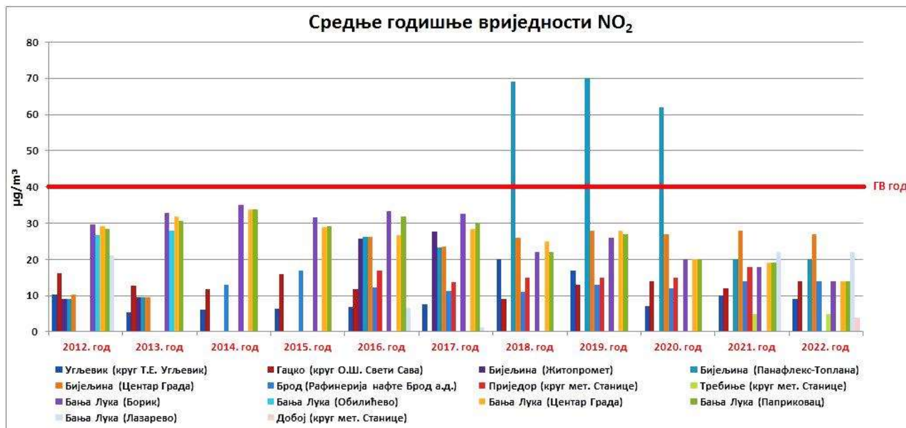
Графикон 9. Упоредни приказ средњих годишњих концентрације NO 2 \mu\text{g}/\text{m}^3 по мјерним мјестима и годинама
