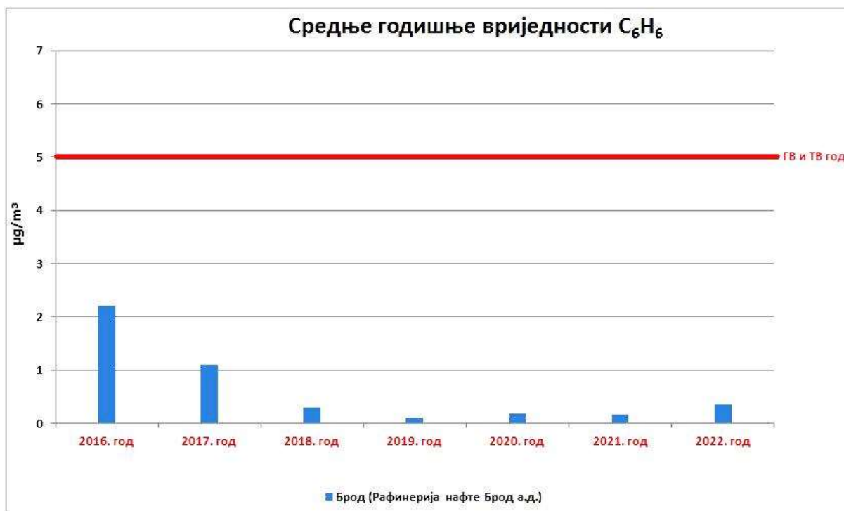
Графикон 49. Упоредни приказ средњих годишњих концентрације C_6H_6 \mu g/m^3 по мјерним мјестима и годинама.
