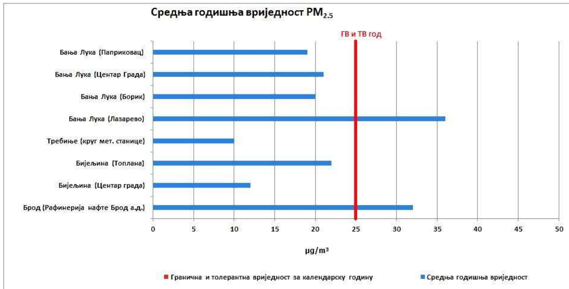
Графикон 24. Упоредни приказ средње годишње концентрације PM_{2.5} \mu g/m^3 по мјерни мјестима у 2022. години.
