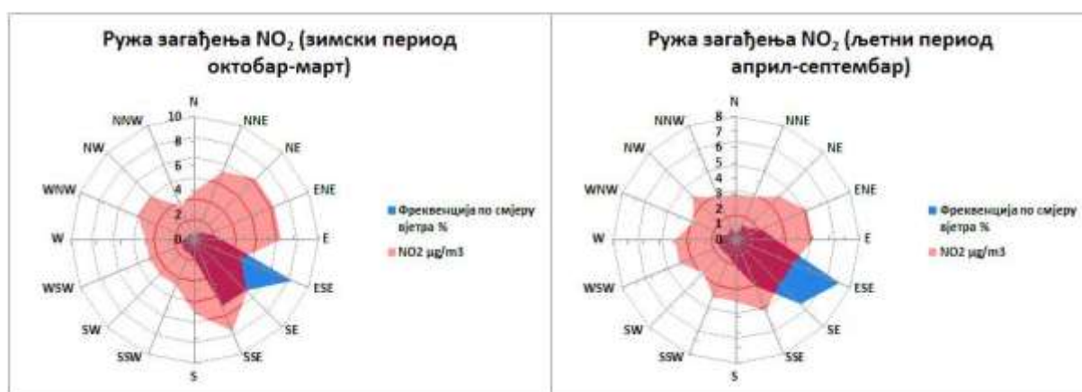
Графикон 15. Руже загађења \text{NO}_2 \mu\text{g}/\text{m}^3 Требиње М.М. круг мет. станице 2022. године
