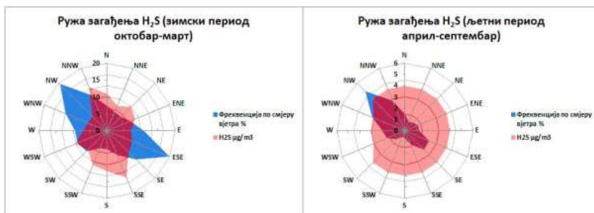
Графикон 47. Руже загађења \text{H}_2\text{S} \mu\text{g}/\text{m}^3 Брод М.М. Рафинерија нафте Брод а.д. 2022. године
