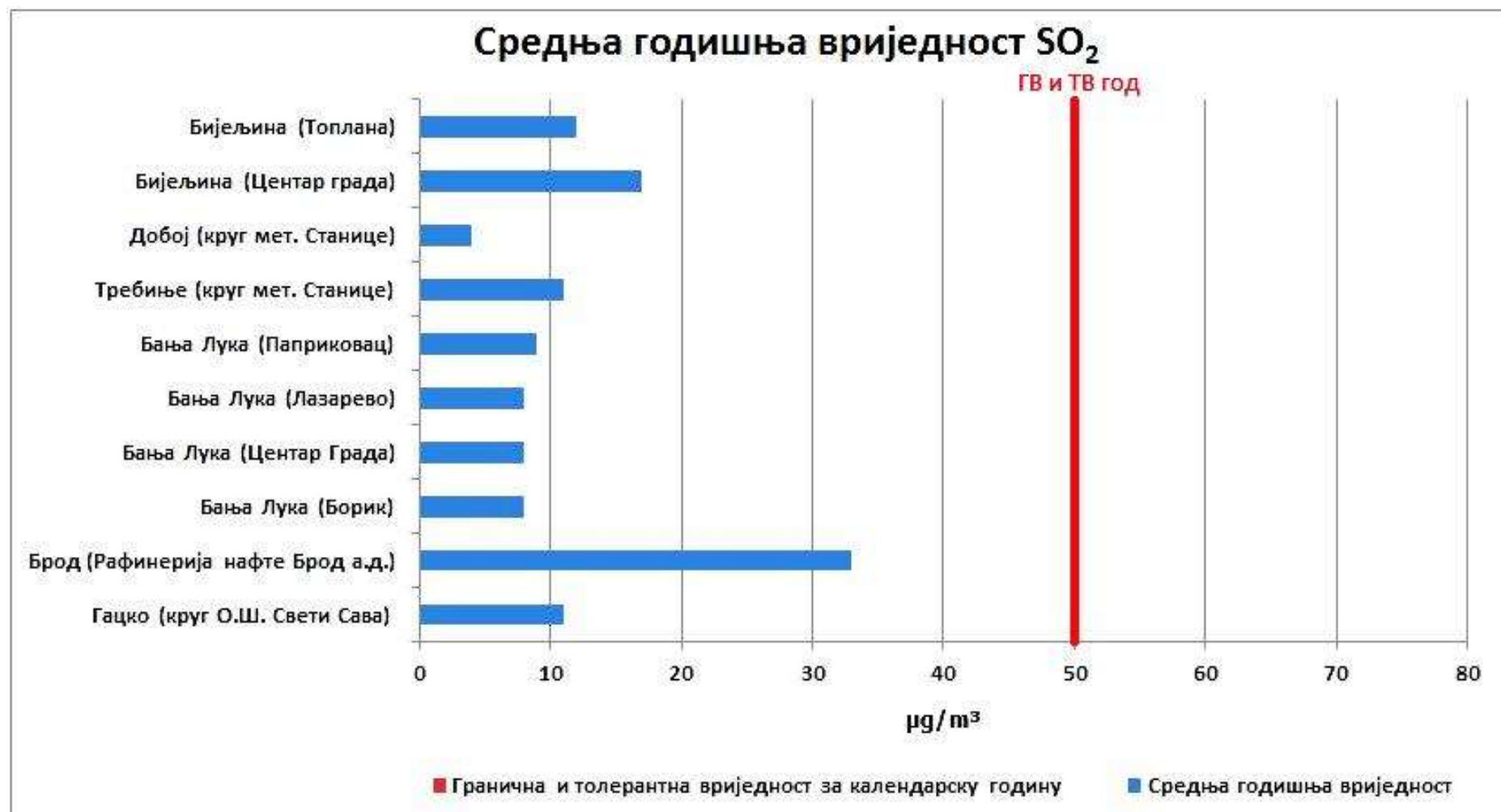
Графикон 1. Упоредни приказ средње годишње концентрације SO 2 µg/m³ по мјерним мјестима у 2022. години.
