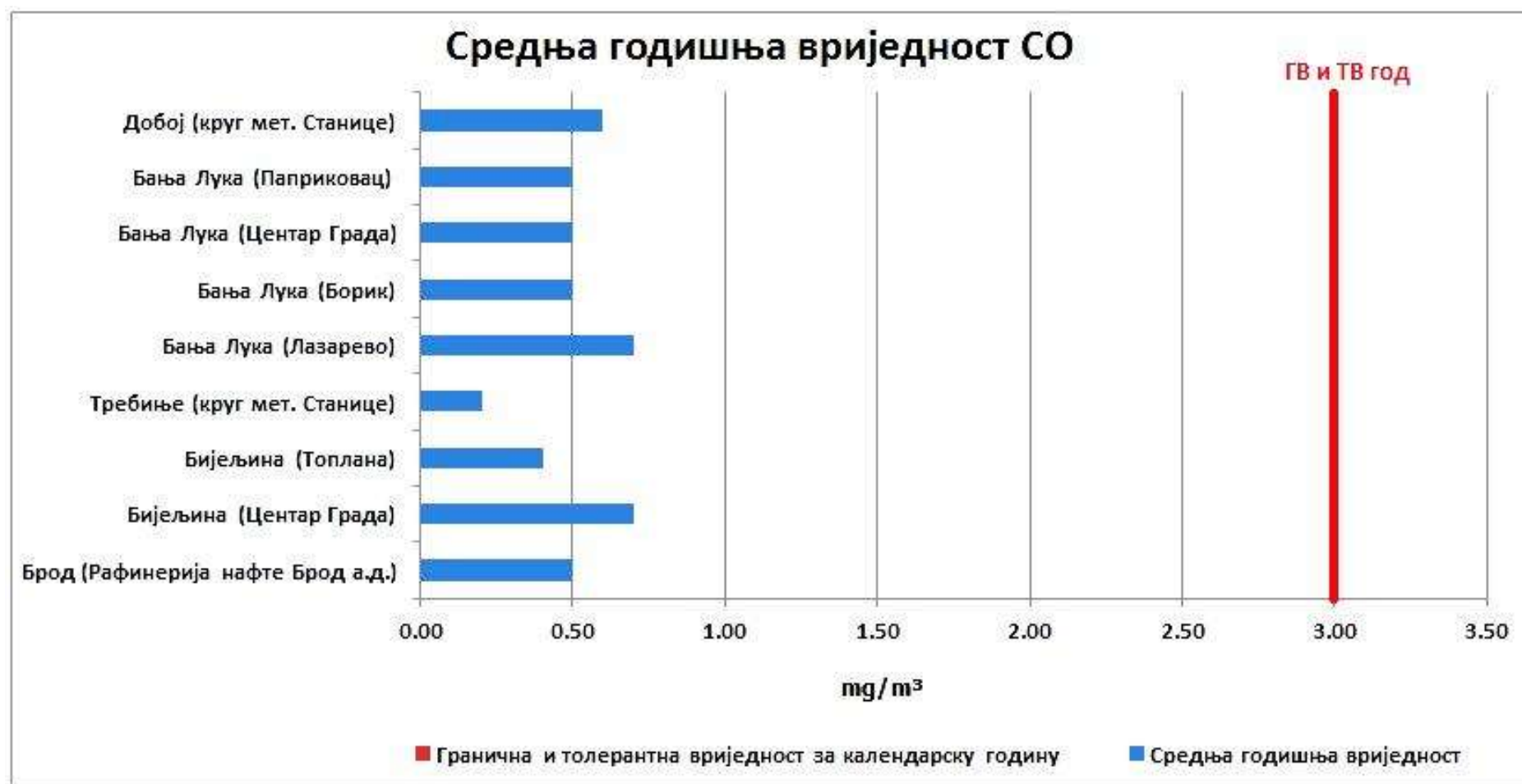
Графикон 29. Упоредни приказ средње годишње концентрације CO mg/m³ по мјерним мјестима у 2022. години
