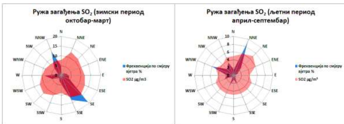
Графикон 6. Руже загађења SO 2 µg/m 3 Бања Лука М.М Лазарево 2022. године
