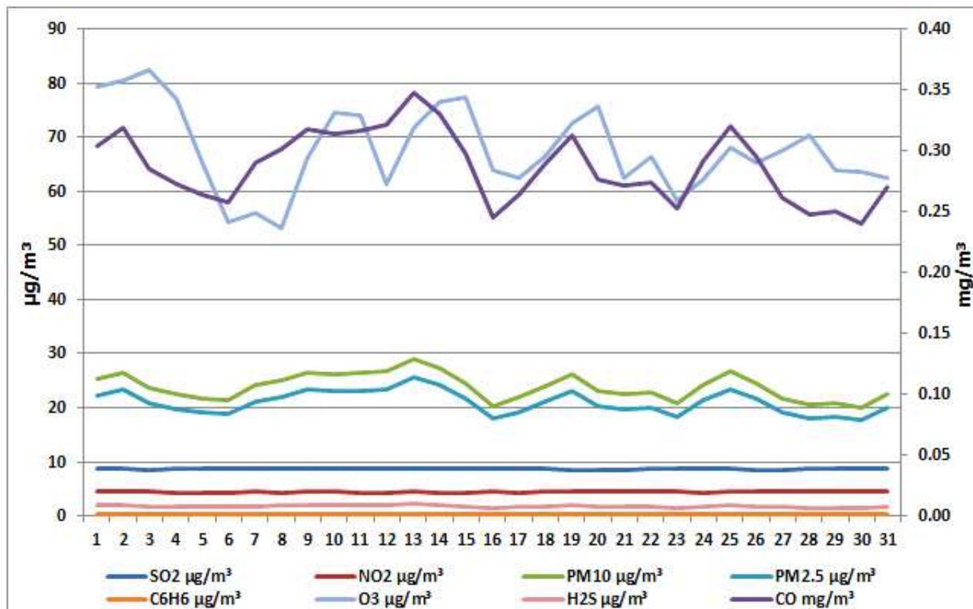
Дијаграм 7. Графички приказ просјечних имисијских дневних концентрација SO 2 , CO, O 3 , C 6 H 6 , H 2 S, NO 2 , PM 2.5 , и PM 10 честица за мај 2025. у Броду (мјерно мјесто Рафинерија нафте Брод а.д.)
