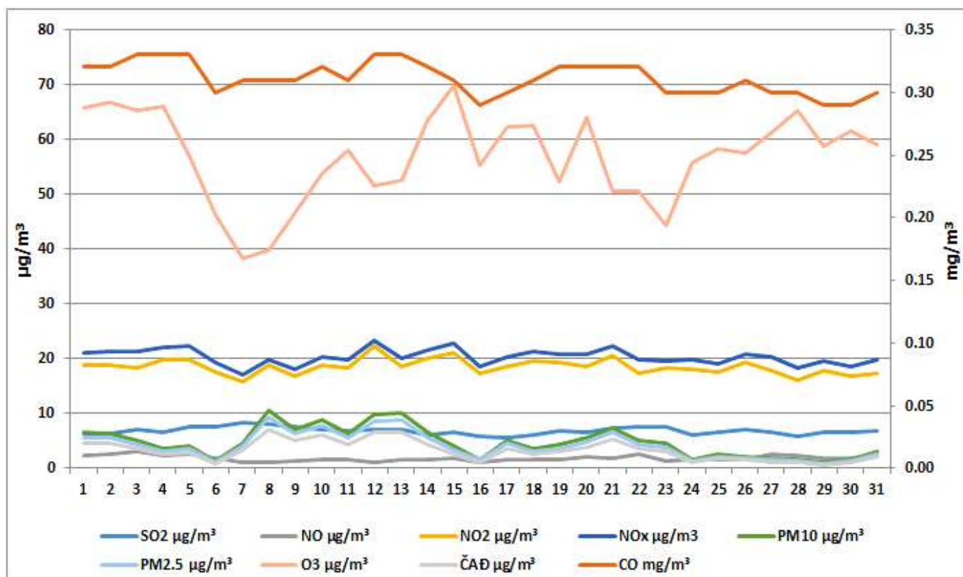
Дијаграм 4. Графички приказ просјечних имисијских дневних SO 2 , CO, NO, NO 2 , NO x , O 3 , ČАД, PM 2.5 и PM 10 за мај 2025. у Бијељини (мјерно мјесто Топлана).
