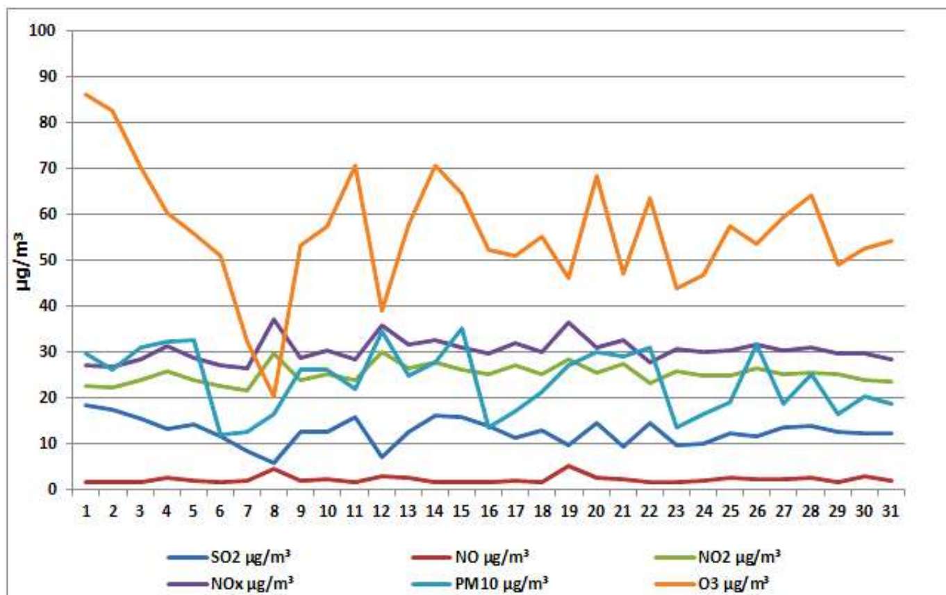
Дијаграм 9. Графички приказ просјечних имисијских дневних концентрација NO, NO 2 , NO x , PM 10 , O 3 и SO 2 за мај 2025. у Добоју (мјерно мјесто круг метеоролошке станице у Добоју)
