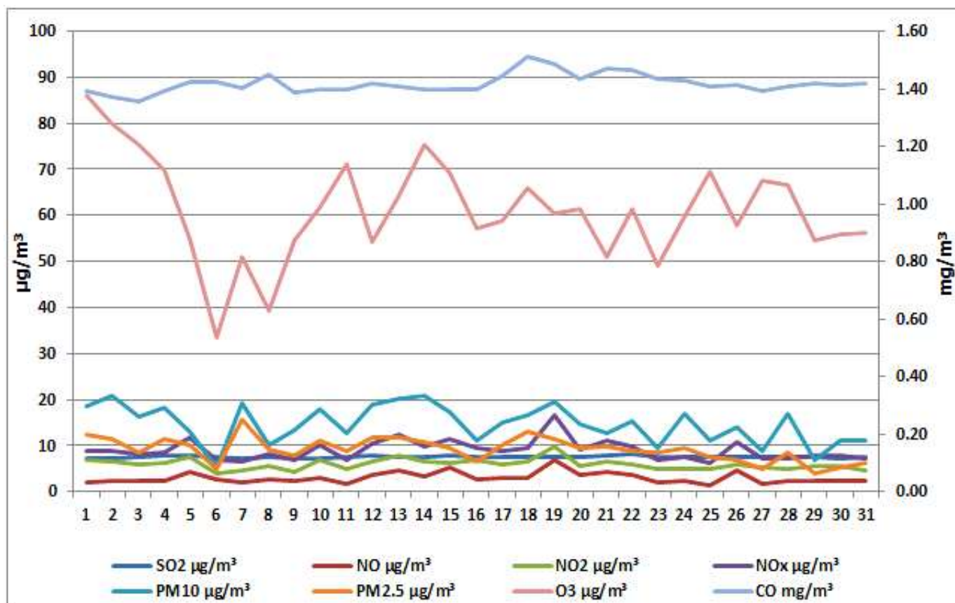
Дијаграм 2. Графички приказ просјечних имисијских дневних концентрација SO 2 , NO, NO 2 , NO x , PM 2.5 , PM 10 , CO и O 3 за мај 2025. у Приједору (мјерно мјесто круг метеоролошке станице у Приједору)
