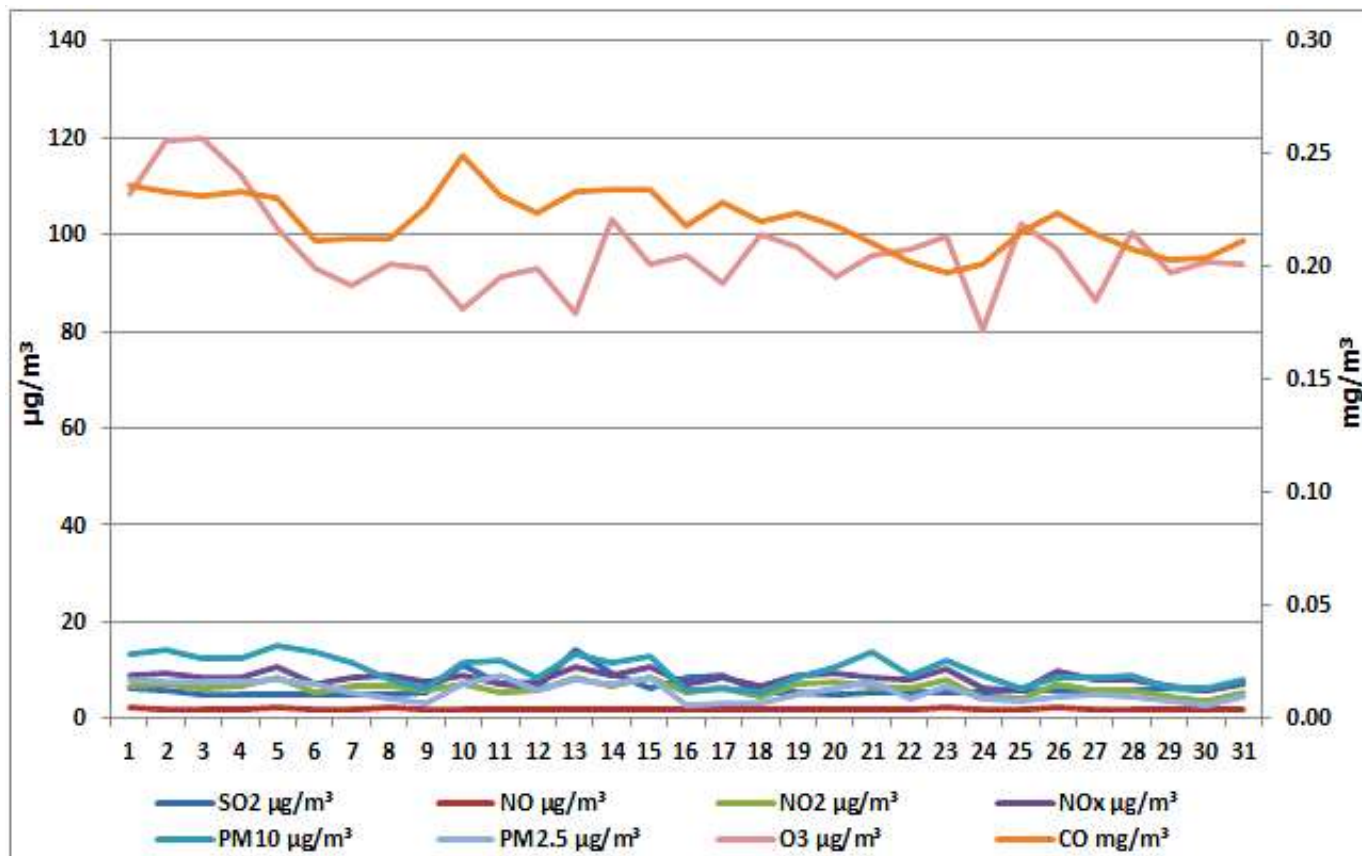
Дијаграм 8. Графички приказ просјечних имисијских дневних концентрација SO 2 , NO, NO 2 , NO x , CO, PM 10 , O 3 и PM 2.5 честица за мај 2025. у Требињу (мјерно мјесто круг метеоролошке станице у Требињу)
