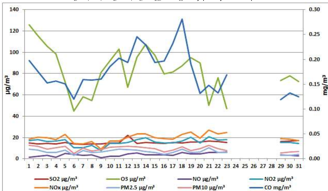
Дијаграм 1. Графички приказ просјечних имисијских дневних концентрација SO 2 , CO, NO, NO 2 , NO x , O 3 , PM 2.5 , и PM 10 за мај 2025 у Бањој Луци (мјерно мјесто Лазарево).
