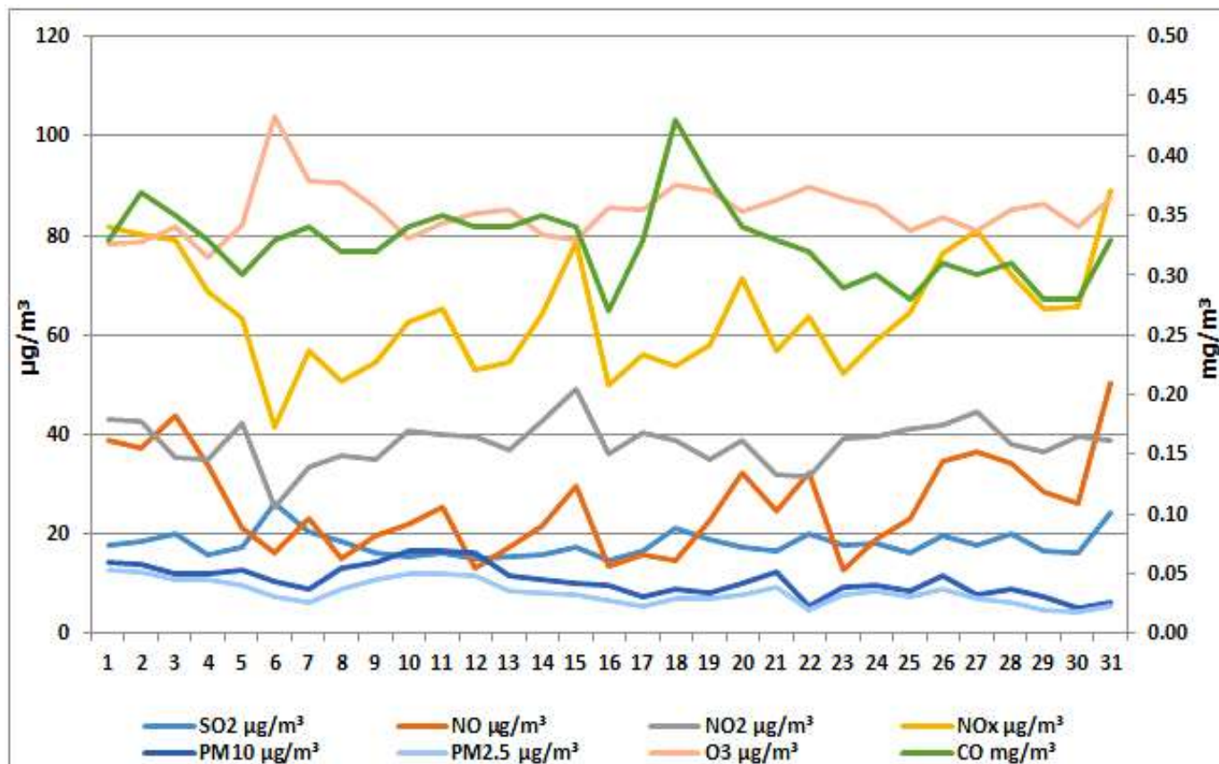
Дијаграм 10. Графички приказ просјечних имисијских дневних концентрација SO 2 , NO, NO 2 , NO x , O 3 , PM 10 , PM 2.5 и CO честица за маја 2025. у Градишци на мјерном мјесту „Црвене зграде“.
