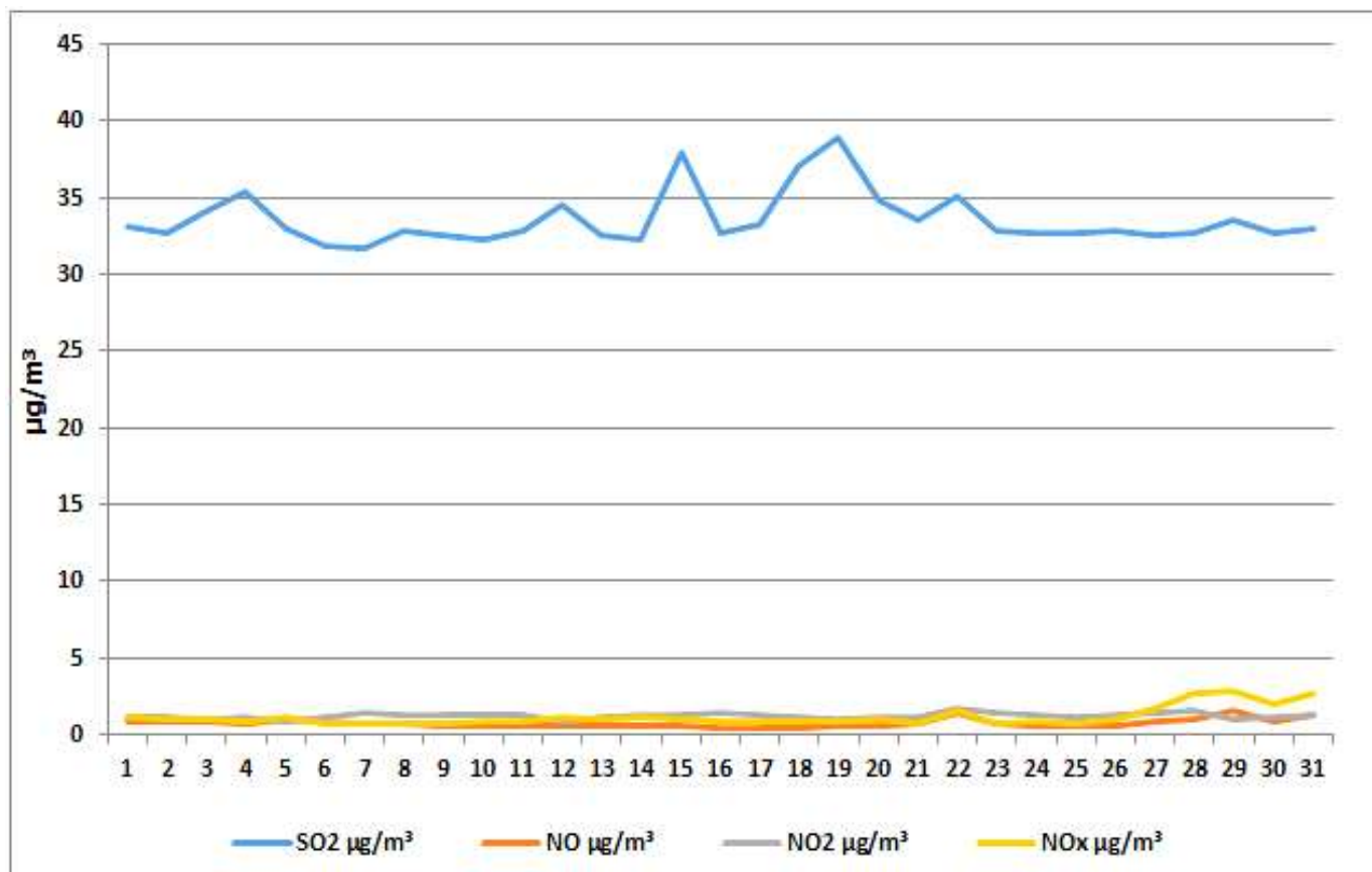
Дијаграм 6. Графички приказ просјечних имисијских дневних концентрација \text{SO}_2 , \text{NO} , \text{NO}_2 , \text{NO}_x и \text{PM}_{10} честица за мај 2025. у Угљевику на мјерном мјесту-круг Т.Е.Угљевик.
