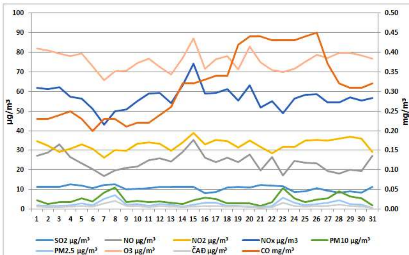
Дијаграм 3. Графички приказ просјечних имисијских дневних SO 2 , CO, NO, NO 2 , NO x , O 3 , ČАД, PM 2.5 и PM 10 за мај 2025. у Бијељини (мјерно мјесто Центар града)
