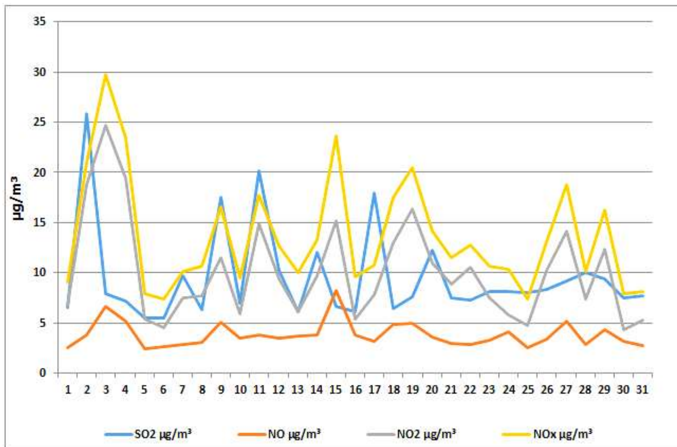
Дијаграм 5. Графички приказ просјечних имисијских дневних концентрација \text{SO}_2 , \text{NO} , \text{NO}_2 и \text{NOx} за мај 2025. у Гацку (мјерном мјесту круг ОШ „Свети Сава“).
