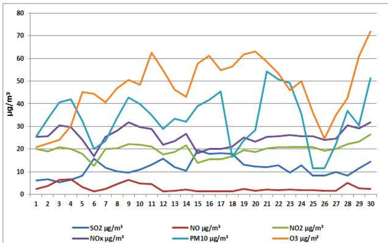
Дијаграм 12. Графички приказ просјечних имисијских дневних концентрација NO, NO 2 , NO x , PM 10 , O 3 и SO 2 за април 2025. у Добоју (мјерно мјесто круг метеоролошке станице у Добоју)
