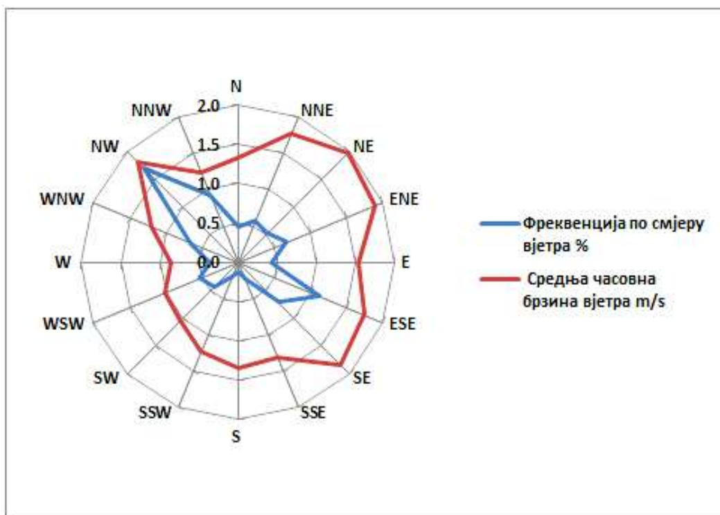
Слика 4. Приказ честине вјетра за април 2025. године у Броду (мјерно мјесто Рафинерија нафте Брод а.д.)
