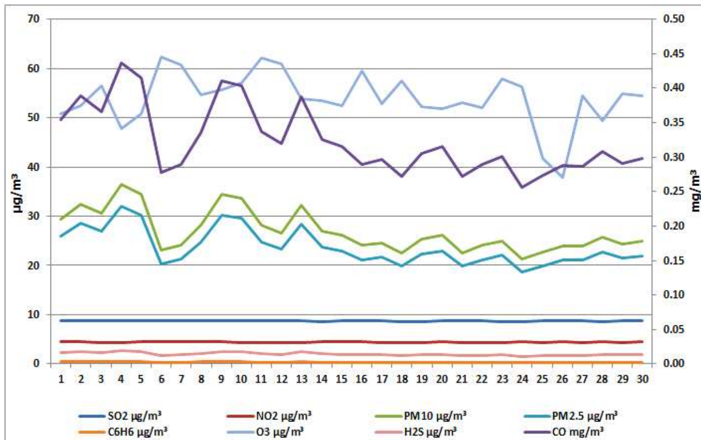
Дијаграм 10. Графички приказ просјечних имисијских дневних концентрација SO 2 , CO, O 3 , C 6 H 6 , H 2 S, NO 2 , PM 2.5 и PM 10 честица за април 2025. у Броду (мјерно мјесто Рафинерија нафте Брод а.д.)
