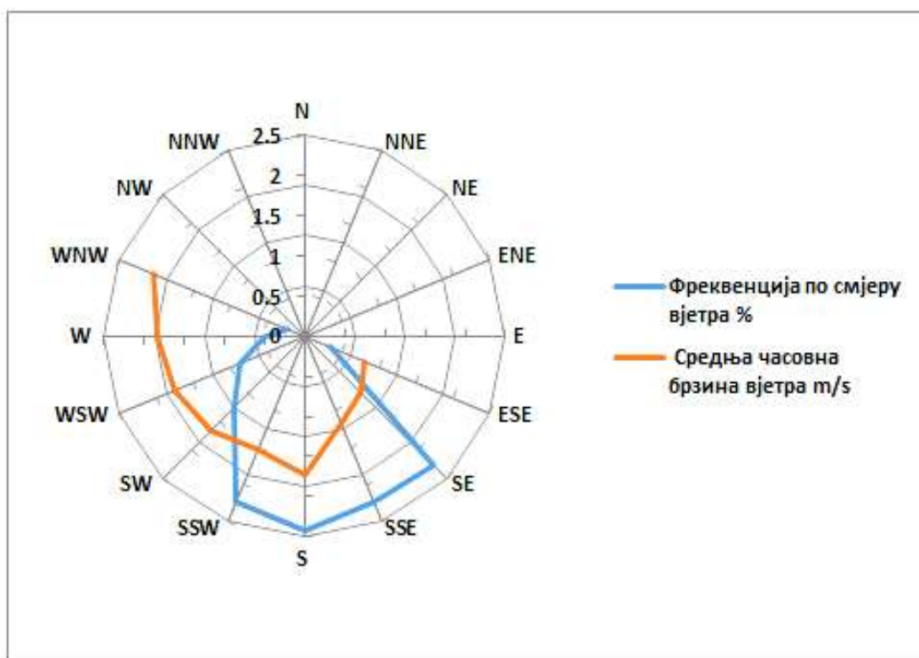
Слика 2. Приказ честине вјетра за април 2025. у Гацку (мјерном мјесту круг ОШ „Свети Сава“).
