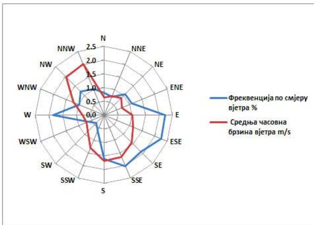
Слика 1. Приказ честине вјетра за април 2025. године у Приједору (мјерно мјесто круг метеоролошке станице у Приједору)
