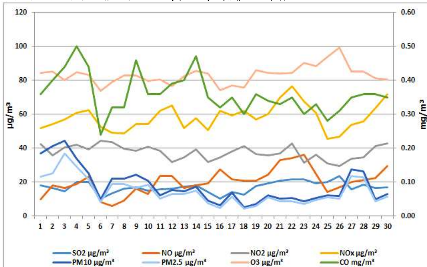
Дијаграм 13. Графички приказ просјечних имисијских дневних концентрација SO 2 , NO, NO 2 , NO x , O 3 , PM 10 , PM 2.5 и CO честица за април 2025. у Градишци на мјерном мјесту „Црвене зграде“.
