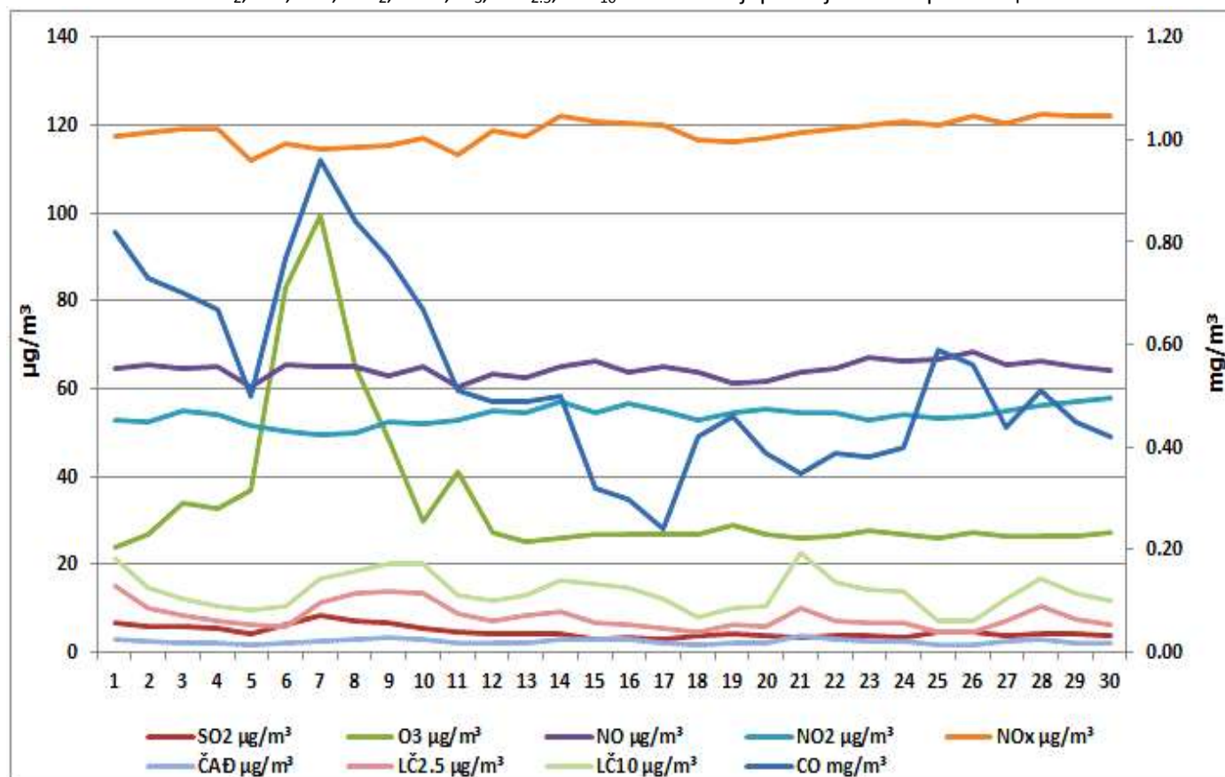
Дијаграм 2. Графички приказ просјечних имисијских дневних концентрација SO 2 , CO, NO, NO 2 , NO x , O 3 , PM 2.5 , PM 10 и ЧАД за април 2025. у Бањој Луци (мјерно мјесто Паприковац)
