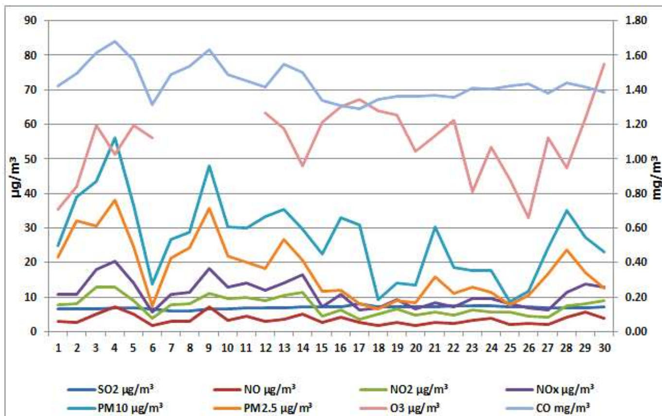
Дијаграм 5. Графички приказ просјечних имисијских дневних концентрација SO 2 , NO, NO 2 , NO x , PM 2.5 , PM 10 , CO и O 3 за април 2025. у Приједору (мјерно мјесто круг метеоролошке станице у Приједору)
