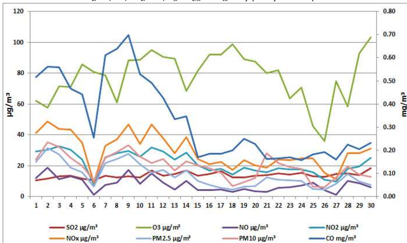
Дијаграм 1. Графички приказ просјечних имисијских дневних концетрација SO 2 , CO, NO, NO 2 , NO x , O 3 , PM 2.5 , и PM 10 за април 2025. у Бањој Луци (мјерно мјесто Лазарево).
