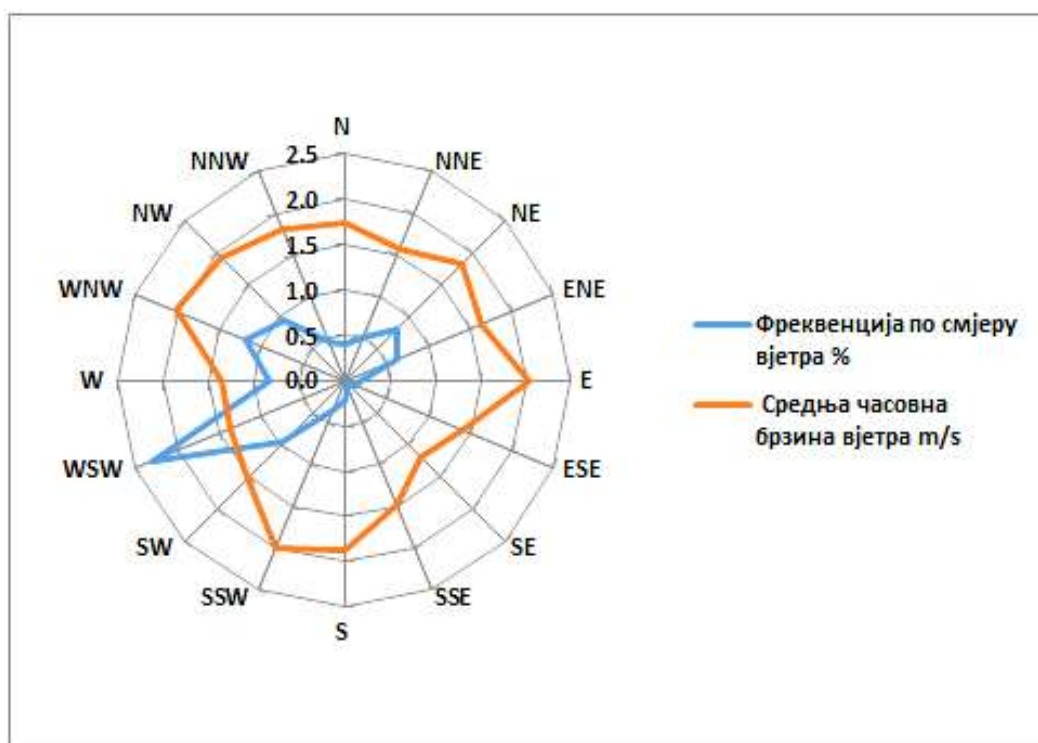
Слика 3. Приказ честине вјетра за април 2025. у Угљевику (мјерном мјесту круг Т.Е.Угљевик).
