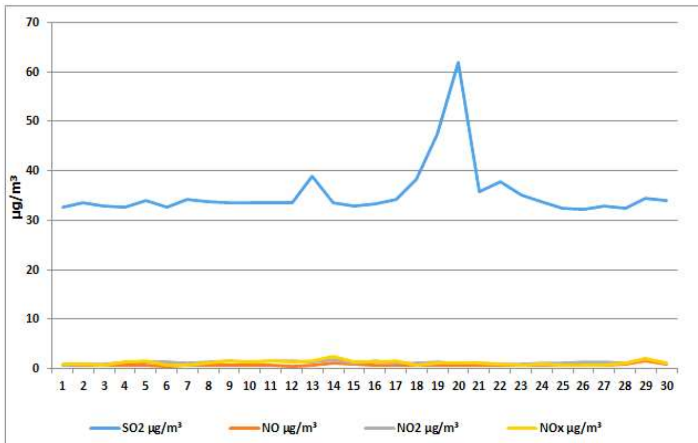
Дијаграм 9. Графички приказ просјечних имисијских дневних концентрација SO 2 , NO, NO 2 и NO x честица за април 2025. у Угљевику на мјерном мјесту-круг Т.Е.Угљевик.
