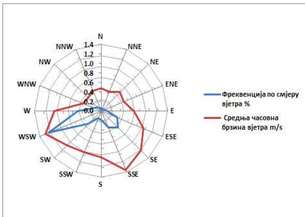
Слика 5. Приказ честине вјетра за април 2025. године у Добоју (мјерно мјесто круг метеоролошке станице у Добоју)
