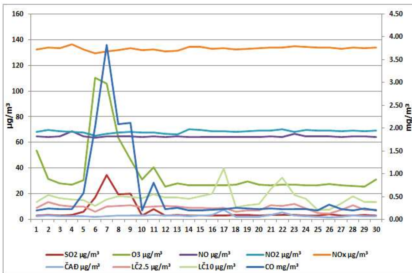
Дијаграм 4. Графички приказ просјечних имисијских дневних концентрација SO 2 , CO, NO, NO 2 , NO x , O 3 , PM 2.5 , PM 10 и ЧАД за април 2025. у Бањој Луци (мјерно мјесто Борик)
