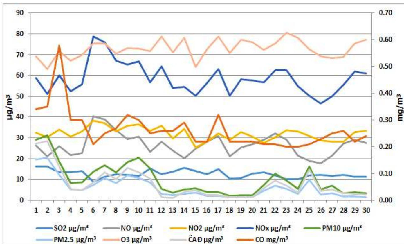
Дијаграм 6. Графички приказ просјечних имисијских дневних SO 2 , CO, NO, NO 2 , NO x , O 3 , ČАД, PM 2.5 и PM 10 за април 2025. у Бијељини (мјерно мјесто Центар града)
