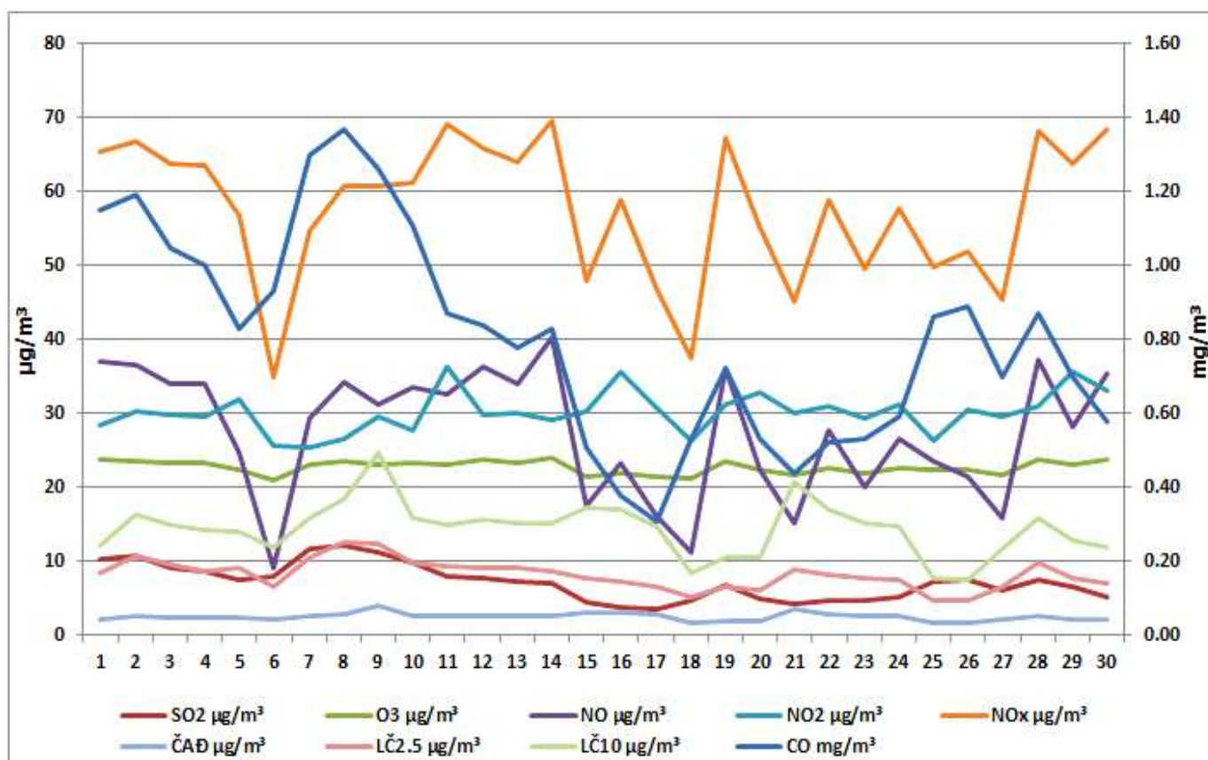
Дијаграм 3. Графички приказ просјечних имисијских дневних концентрација SO 2 , CO, NO, NO 2 , NO x , PM 2.5 , PM 10 , O 3 и ЧАД за април 2025. у Бањој Луци (мјерно мјесто Центар града)
