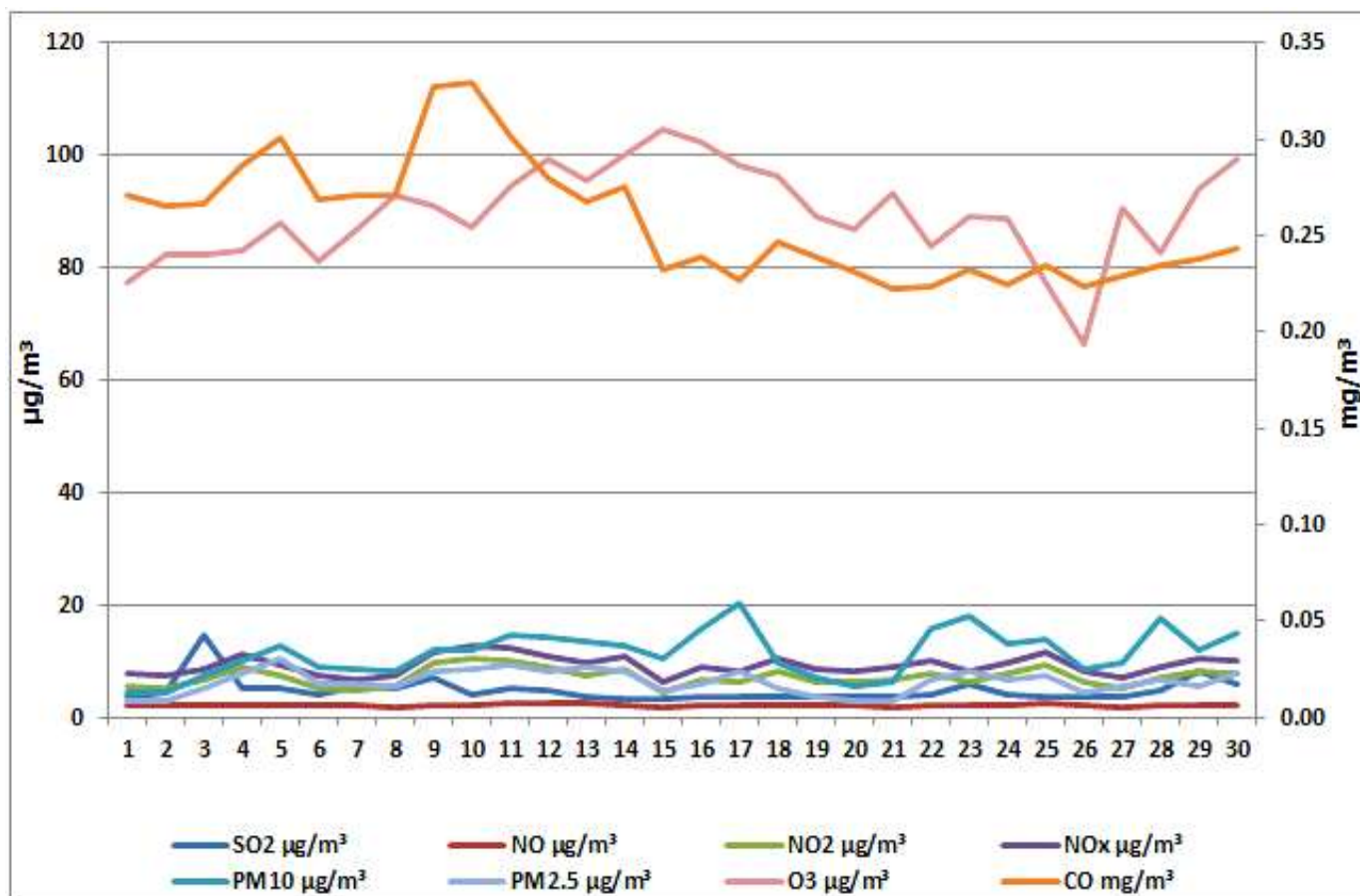
Дијаграм 11. Графички приказ просјечних имисијских дневних концентрација SO 2 , NO, NO 2 , NO x , CO, PM 10 , O 3 и PM 2.5 честица за април 2025. у Требињу (мјерно мјесто круг метеоролошке станице у Требињу)
