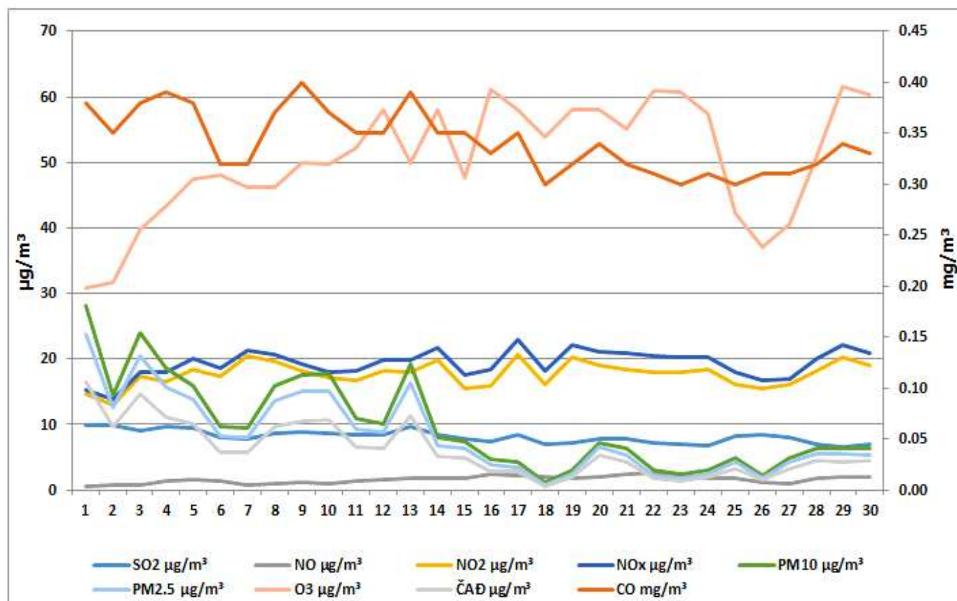
Дијаграм 7. Графички приказ просјечних имисијских дневних SO 2 , CO, NO, NO 2 , NO x , O 3 , ČАД, PM 2.5 и PM 10 за април 2025. у Бијељини (мјерно мјесто Топлана).
