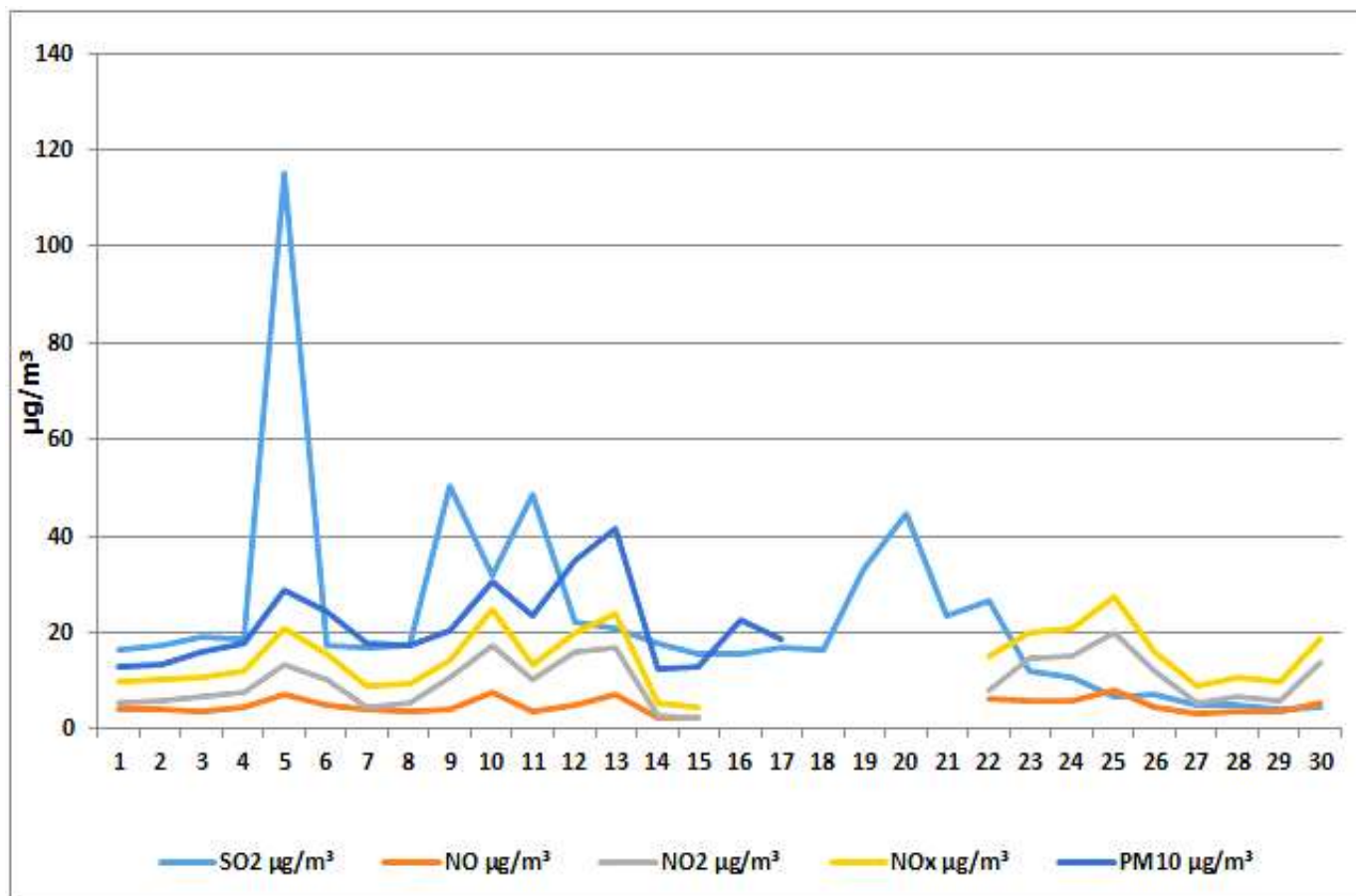
Дијаграм 8. Графички приказ просјечних имисијских дневних концентрација \text{SO}_2 , \text{NO} , \text{NO}_2 , \text{NO}_x , и \text{PM}_{10} за април 2025. у Гацку (мјерном мјесту круг ОШ „Свети Сава“).
